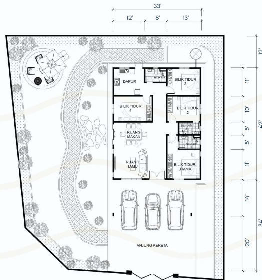
PELAN LANTAI
