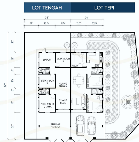
PELAN LANTAI
