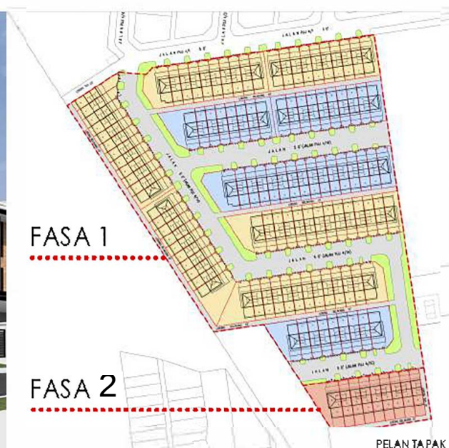
PELAN TAPAK
