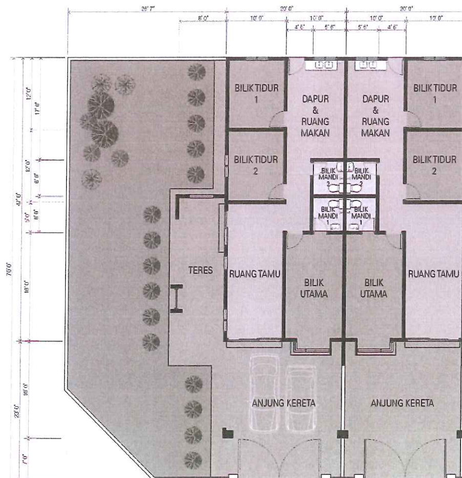
Pelan Lantai
