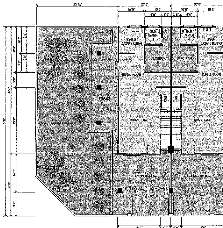
PELAN TINGKAT ATAS
