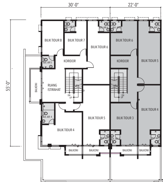
PELAN LANTAI TINGKAT 1
