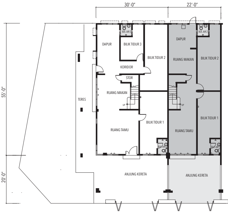
PELAN LANTAI TINGKAT BAWAH
