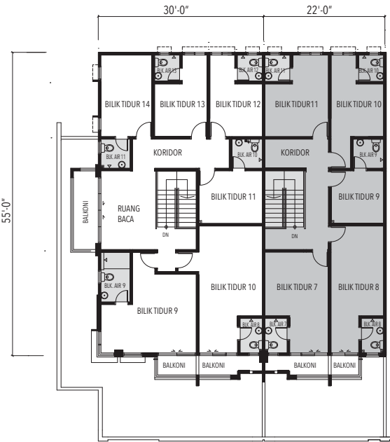
PELAN LANTAI TINGKAT 2
