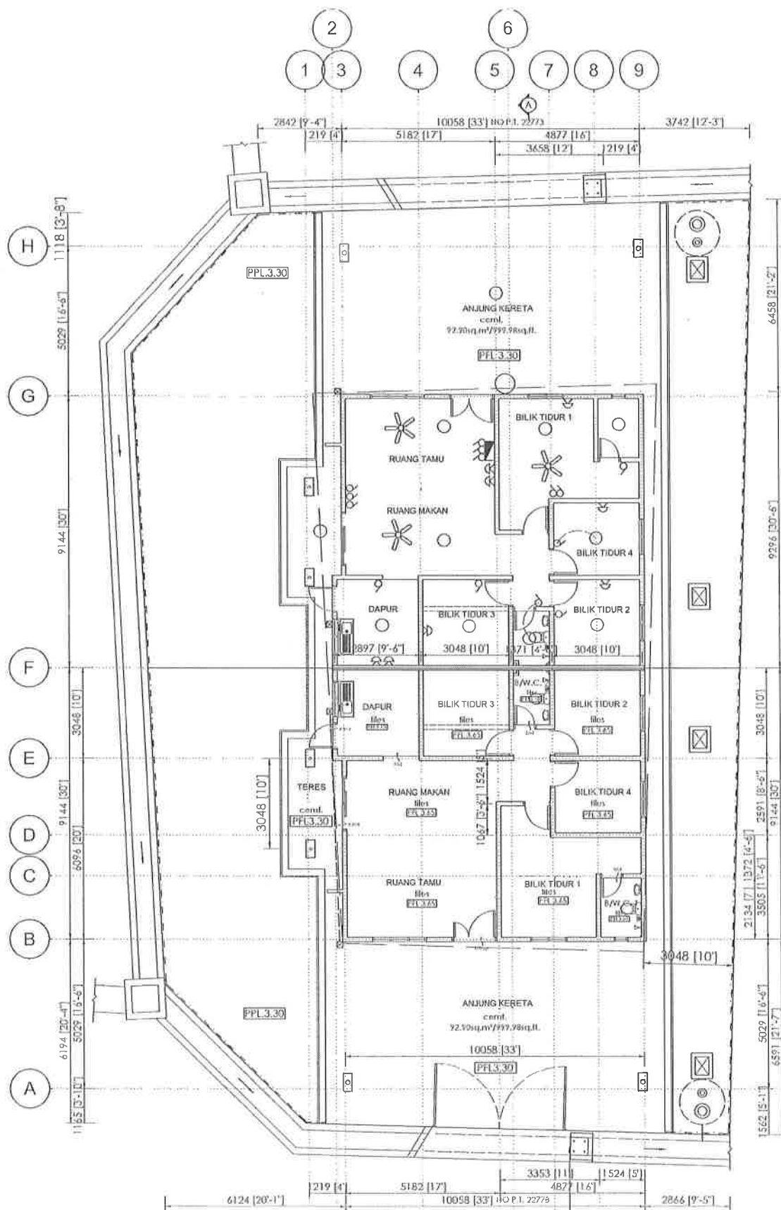
PELAN LANTAI
