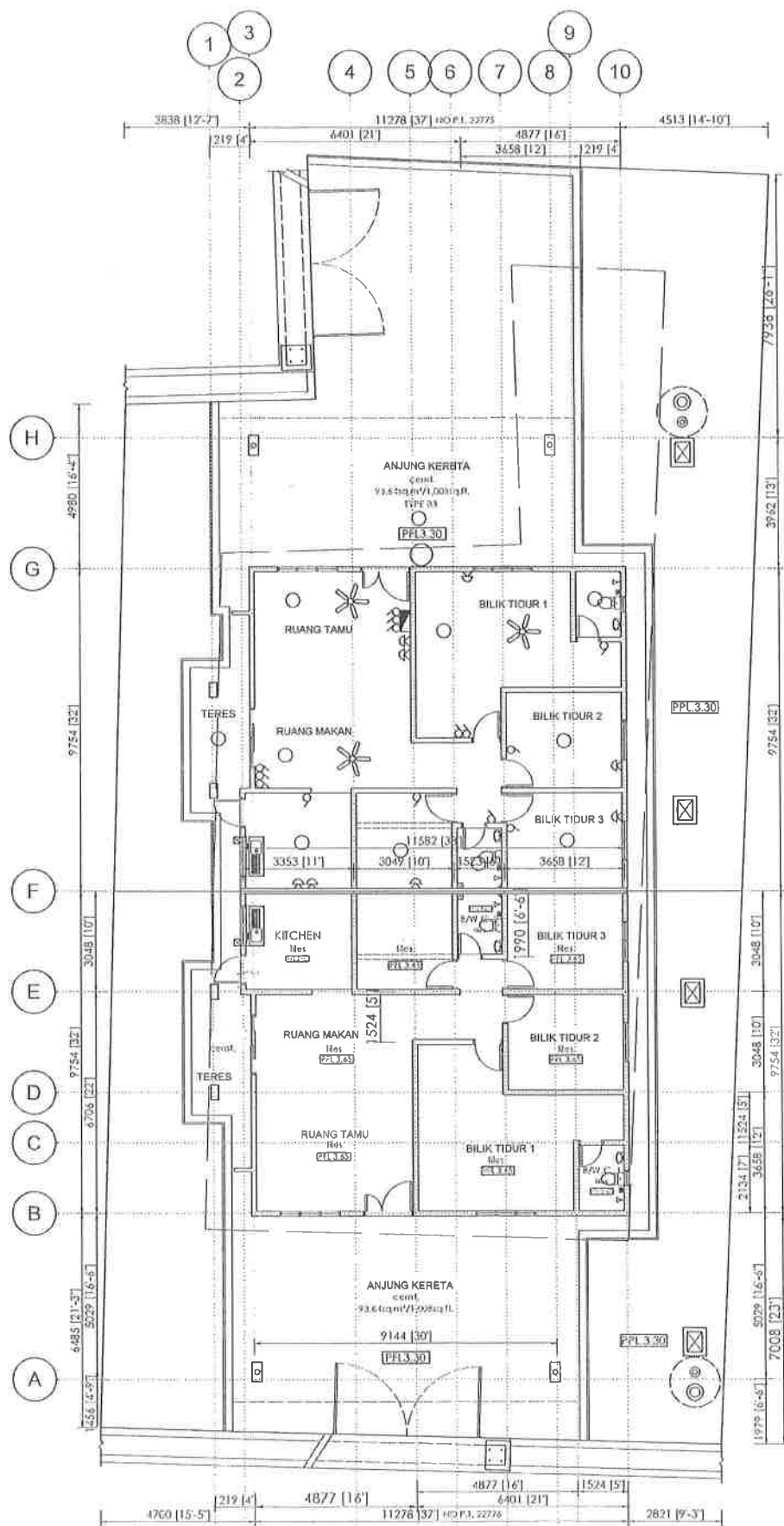
PELAN LANTAI
