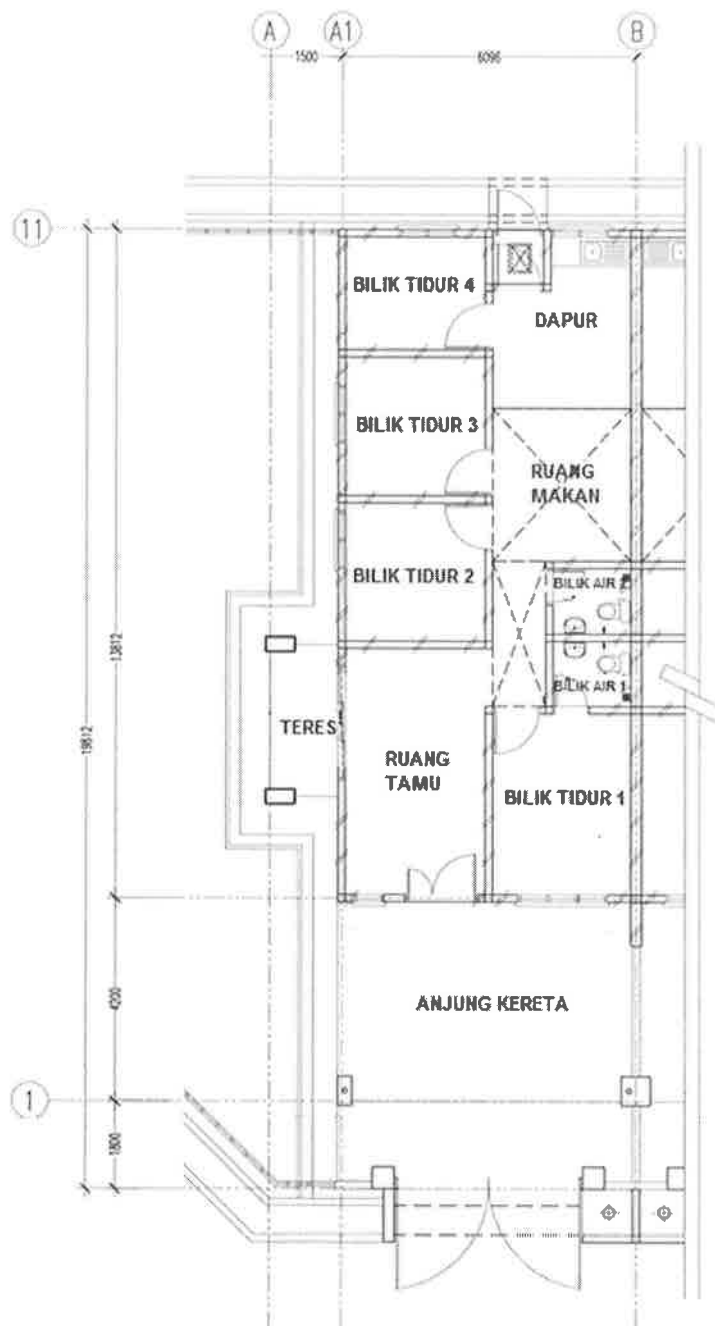
PELAN LANTAI
