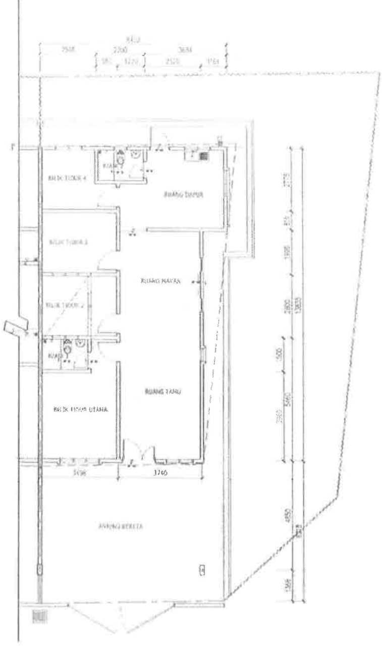
PELAN LANTAI
