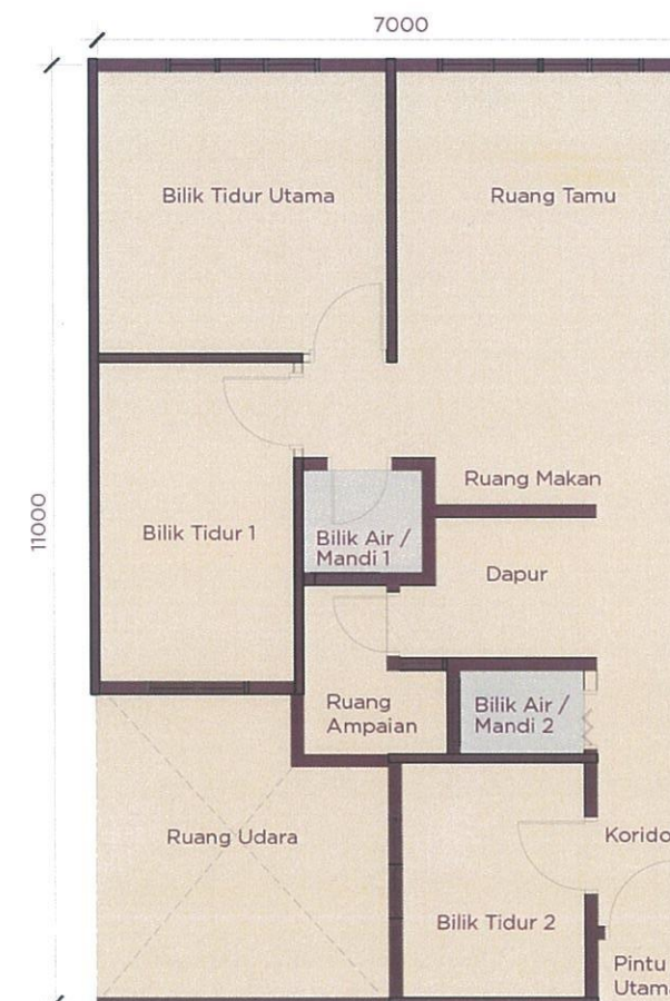
PELAN LANTAI
