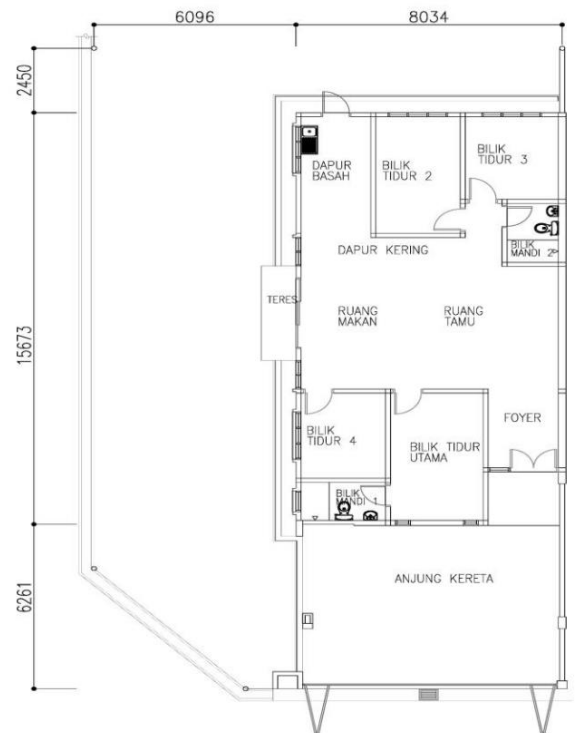
PELAN LANTAI
