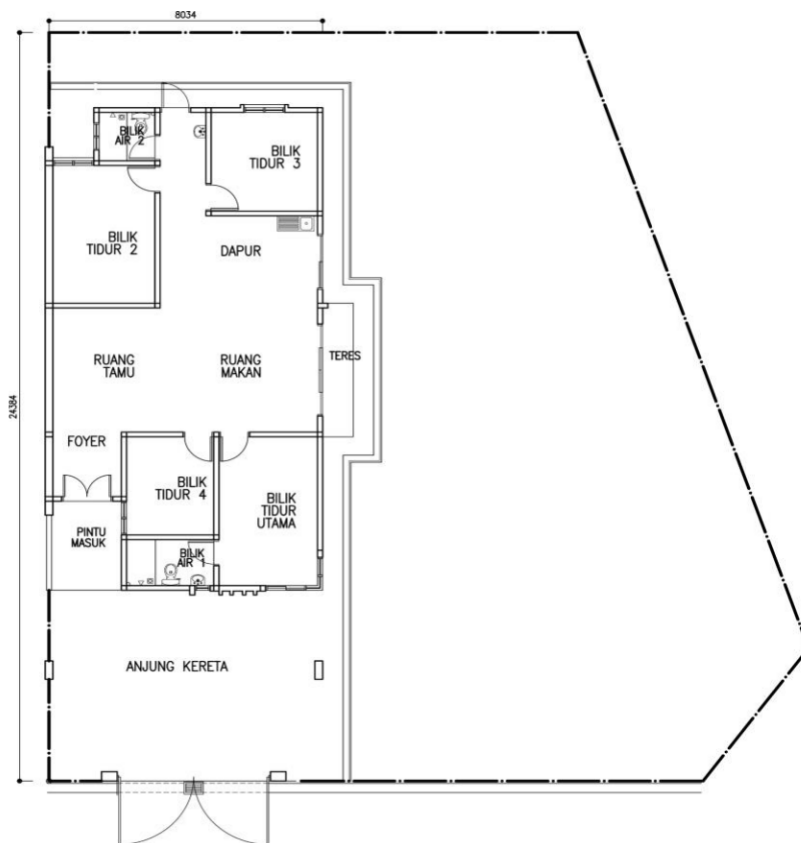
PELAN LANTAI
