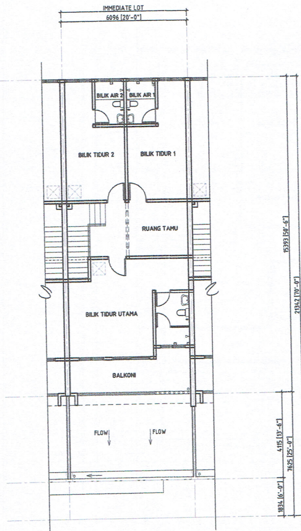
PELAN LANTAI ATAS
