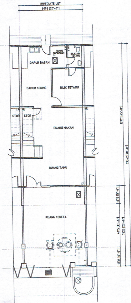
PELAN LANTAI BAWAH
