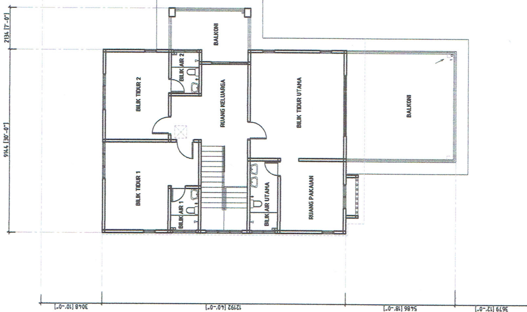
PELAN TINGKAT ATAS
