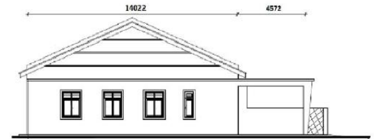
PANDANGAN TEPI
