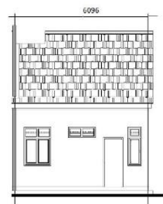
PANDANGAN BELAKANG
