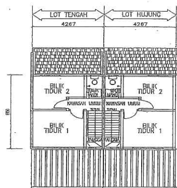
PELAN LANTAI ARAS SATU
