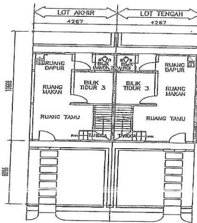
PELAN TAPAK BAWAH
