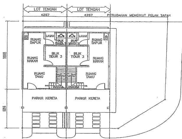
PELAN TAPAK BAWAH
