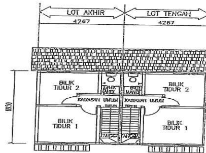
PELAN LANTAI ARAS SATU
