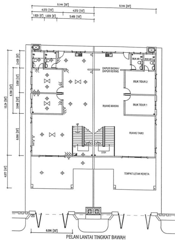
RUMAH BERBANDUNG 2 TINGKAT ( DOUBLE STOREY ) JENIS 'A' ( PTD 29316, PTD 29317, PTD 29318 & PTD 29319 )
