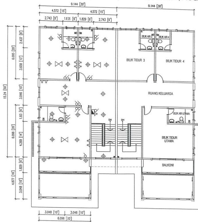
PELAN LANTAI TINGKAT 1
