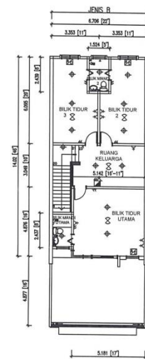
PELAN LANTAI TINGKAT ATAS
