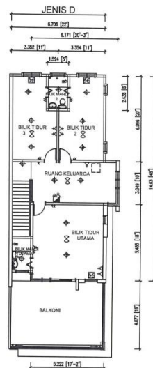
PELAN LANTAI TINGKAT ATAS
