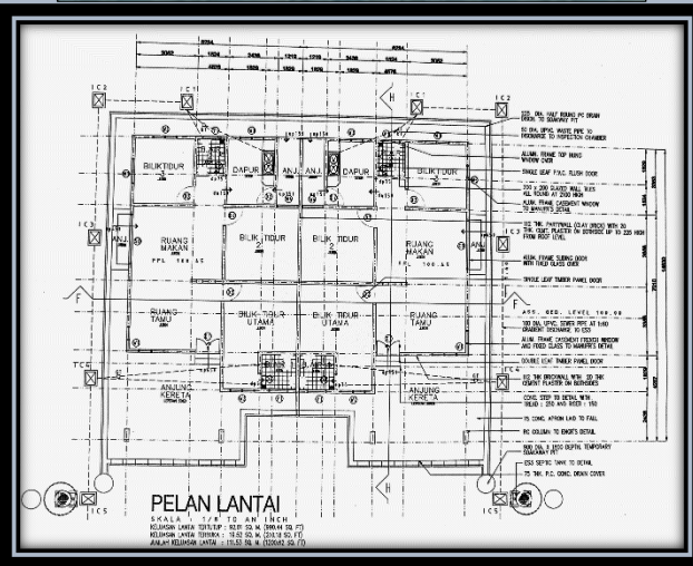
PLAN LANTAI SEMI-D
