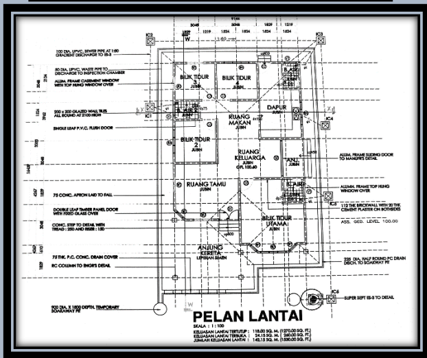
PLAN LANTAI BANGLO JENIS A
