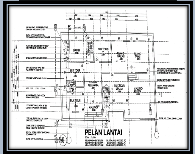
PLAN LANTAI BANGLO JENIS B
