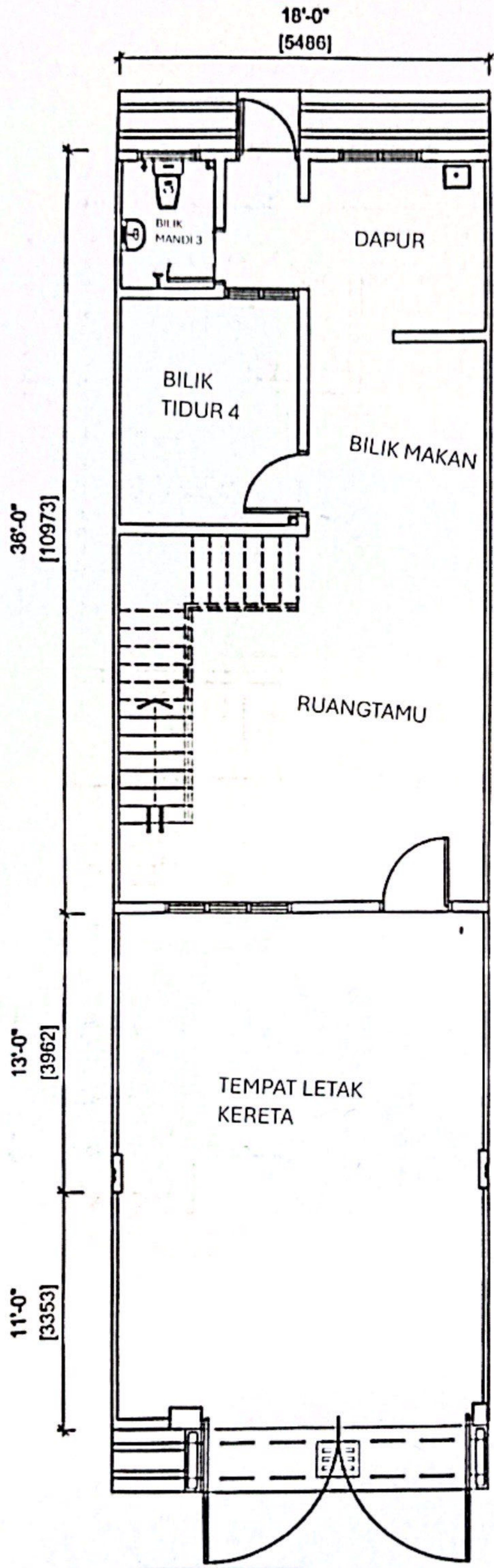
PELAN TINGKAT BAWAH (RUMAH TERES)
