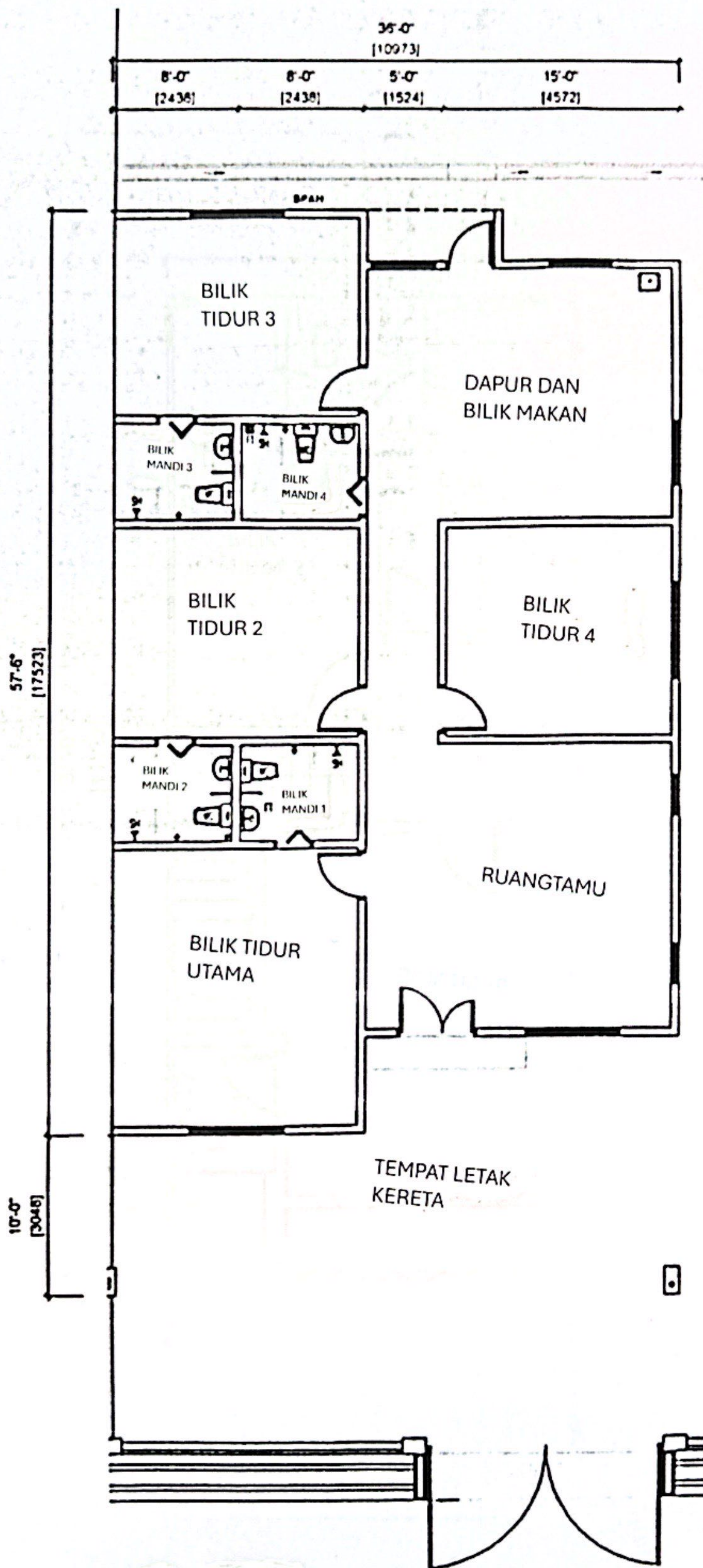
PELAN TINGKAT BAWAH (RUMAH BERKEMBAR)
