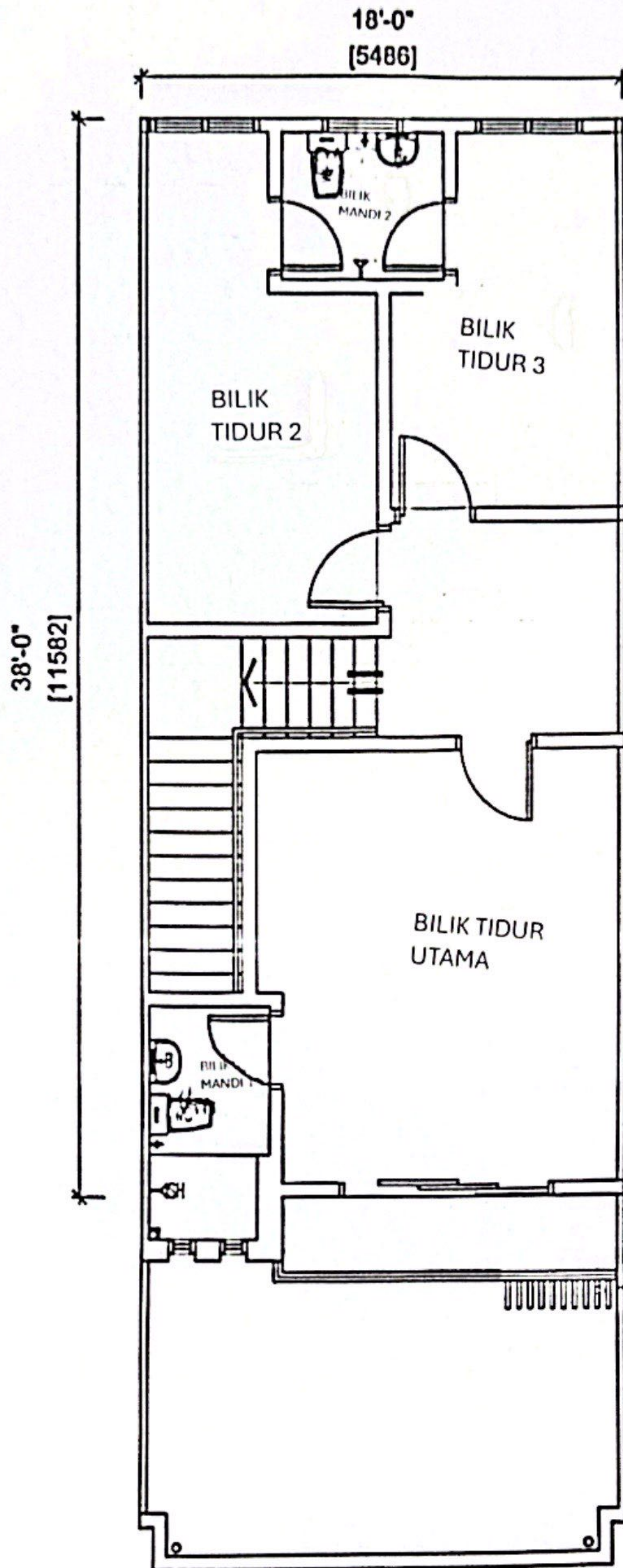
PELAN TINGKAT SATU (RUMAH TERES)
