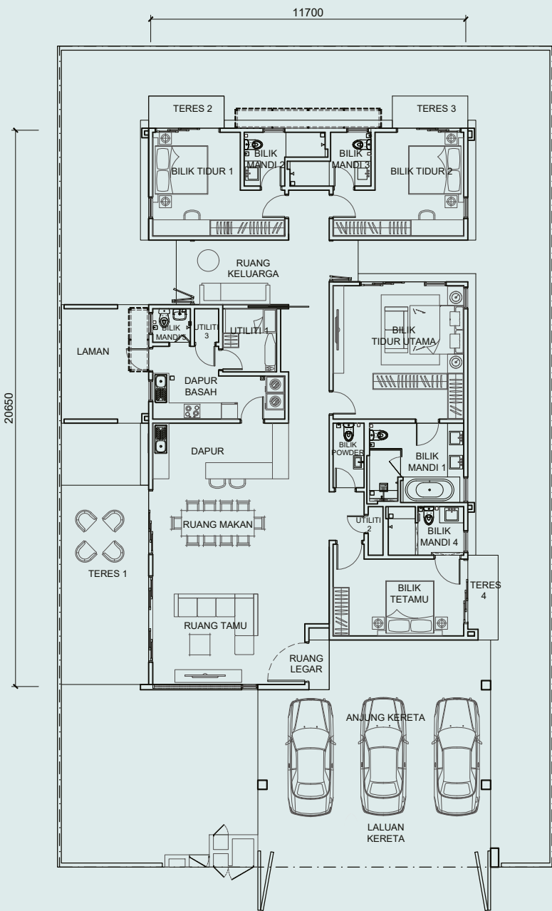
TINGKAT BAWAH
