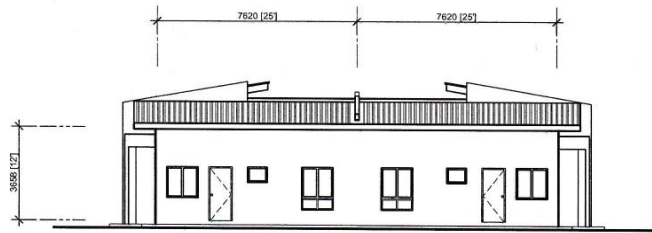
PANDANGAN BELAKANG
