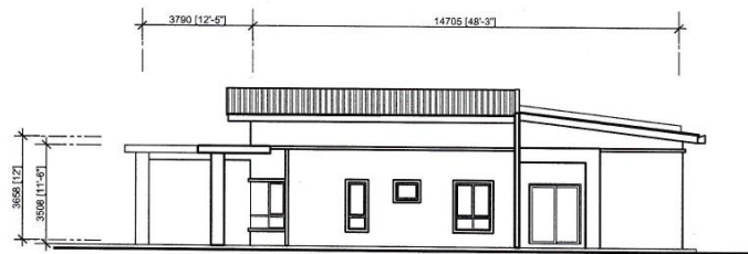
PANDANGAN KANA
