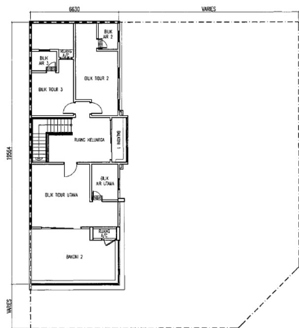
PELAN LANTAI ARAS SATU
