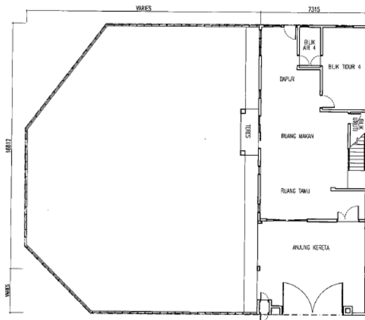
PELAN LANTAI ARAS TANAH
