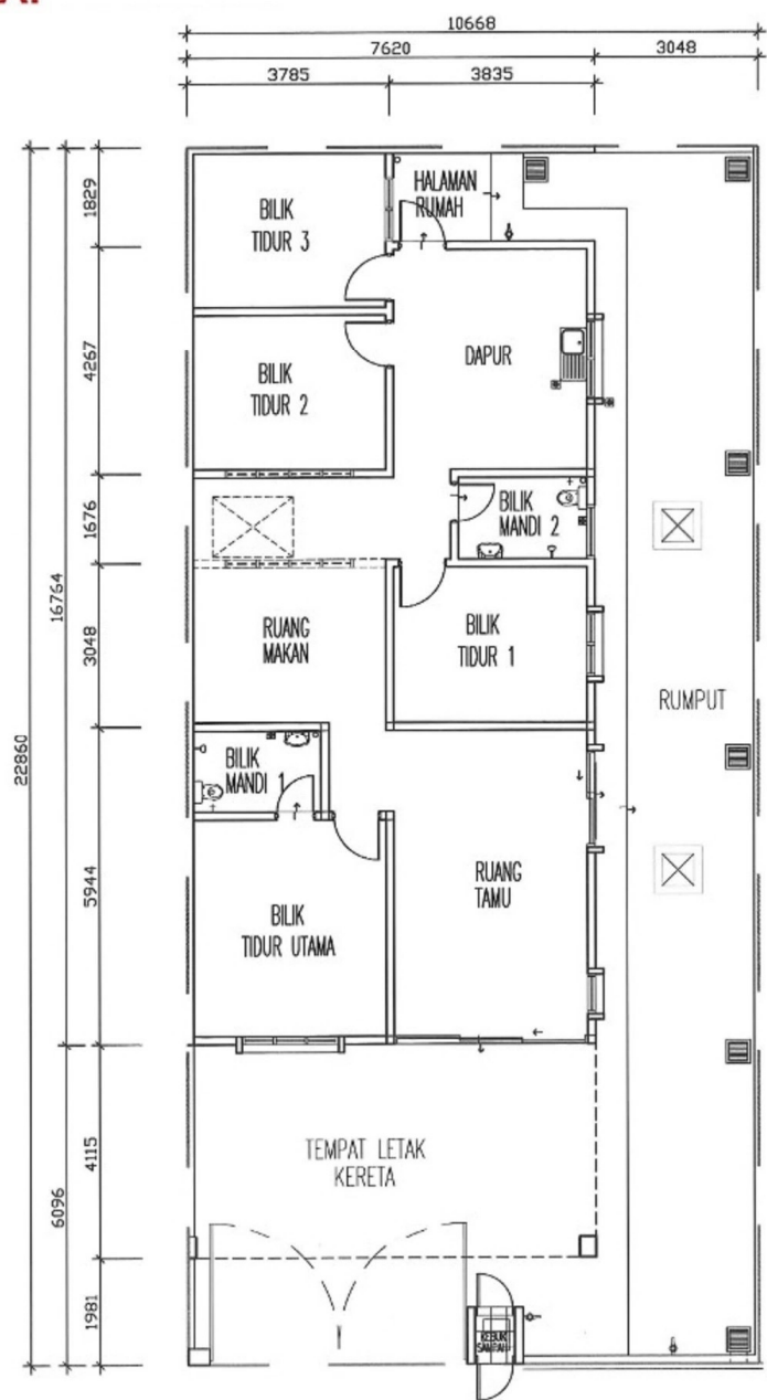
PELAN TINGKAT BAWAH
