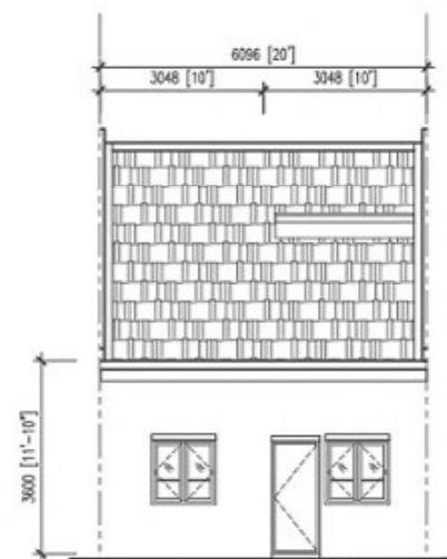
PANDANGAN BELAKANG
