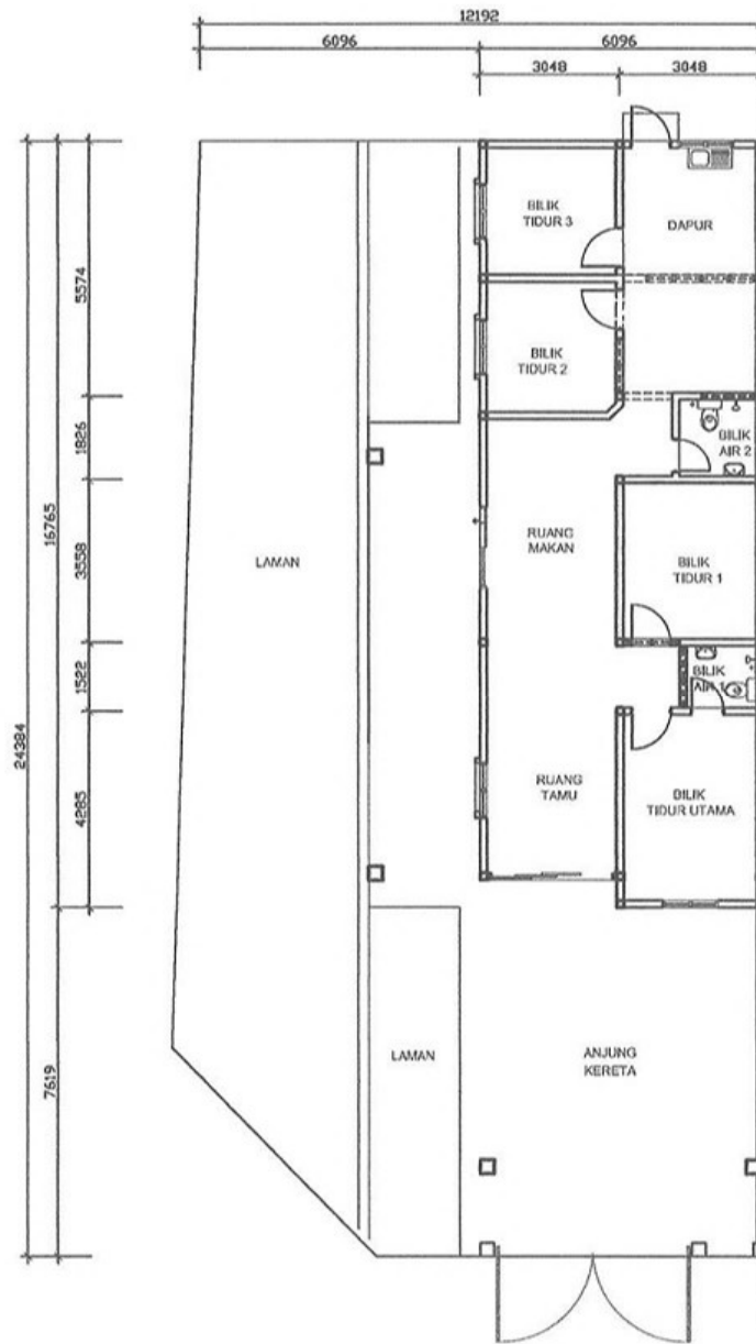
PELAN TINGKAT BAWAH
