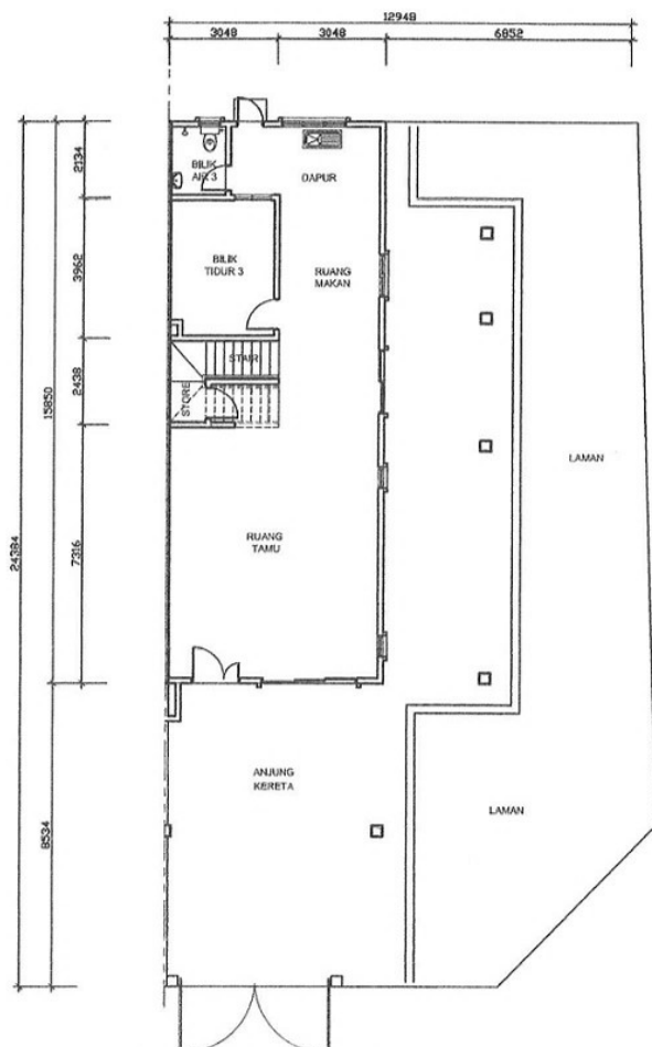
PELAN TINGKAT BAWAH
