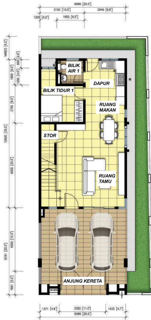
TINGKAT BAWAH 1 : 100
