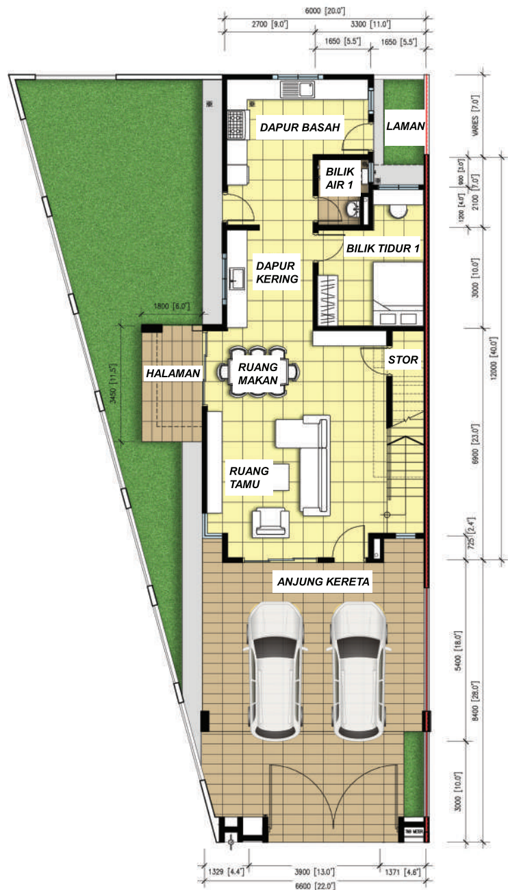
TINGKAT BAWAH
