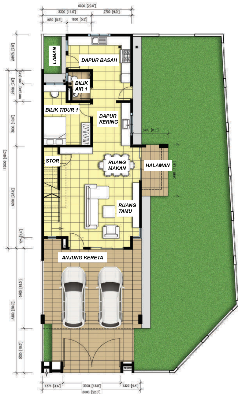
TINGKAT BAWAH 1:100
