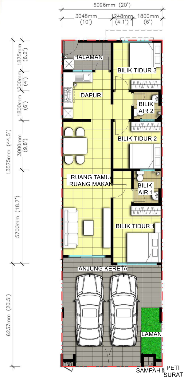
RUMAH TERES 1 TINGKAT - TENGAH
