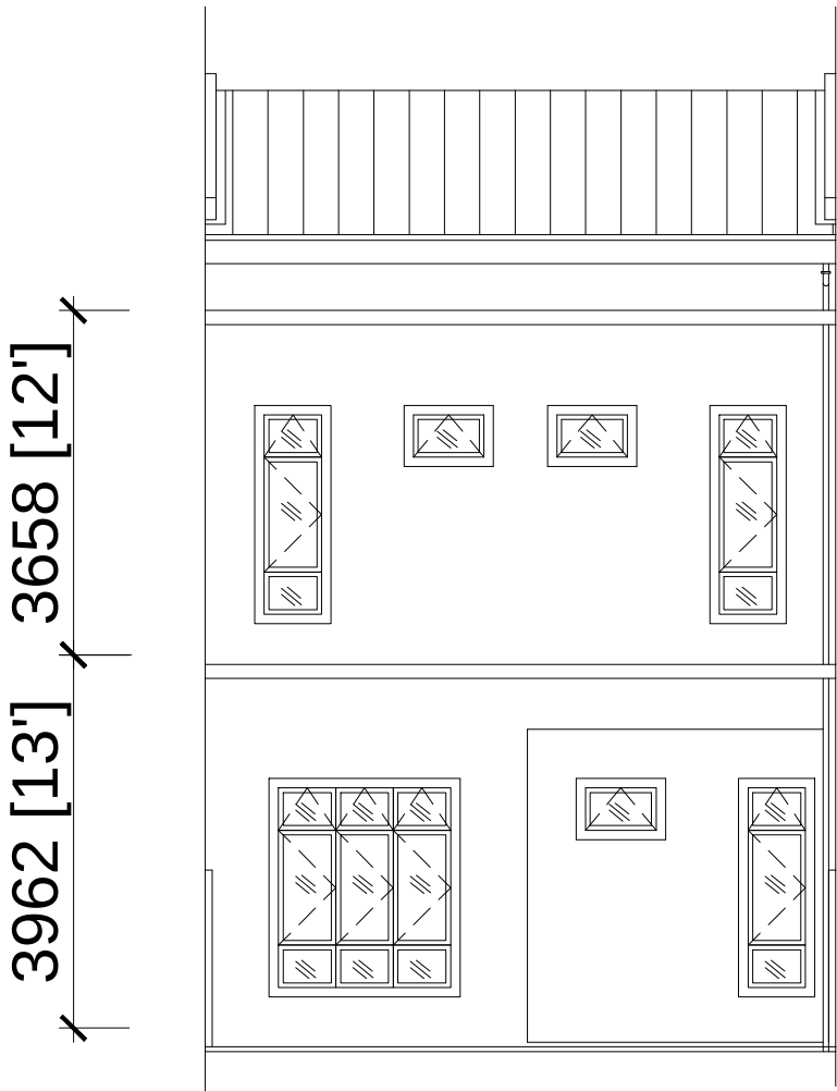
PANDANGAN BELAKANG RUMAH TERES 2 TINGKAT - TYPE B (PTD.4709,PTD.4711,PTD.4713,PTD.4715,PTD.4717,PTD.4719, PTD.4724,PTD.4726,PTD.4728,PTD.4730,PTD.4732,PTD.4734)
