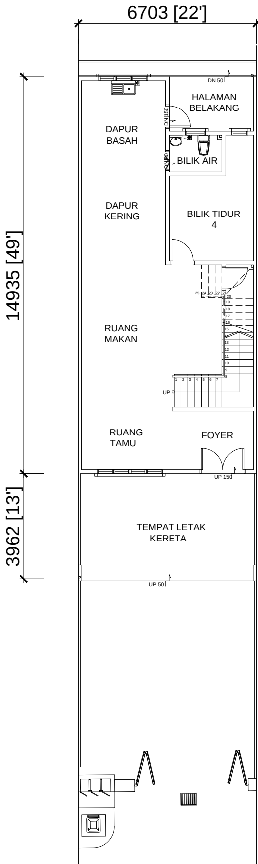
PELAN LANTAI BAWAH RUMAH TERES 2 TINGKAT - TYPE B (PTD.4709,PTD.4711,PTD.4713,PTD.4715,PTD.4717,PTD.4719, PTD.4724,PTD.4726,PTD.4728,PTD.4730,PTD.4732,PTD.4734)
