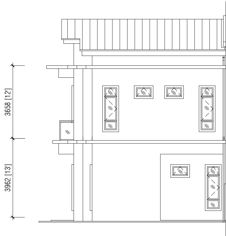
PANDANGAN BELAKANG RUMAH TERES 2 TINGKAT - TYPE D (PTD. 4707)
