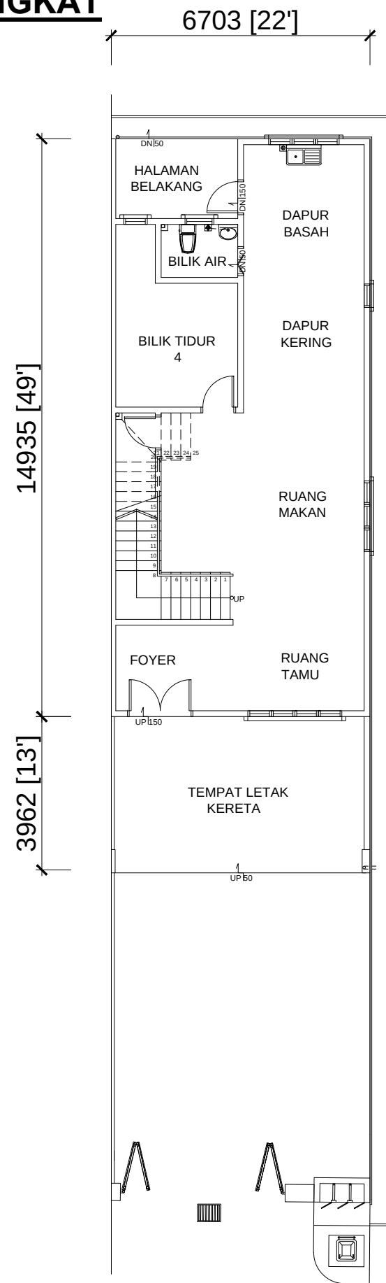
PELAN LANTAI BAWAH RUMAH TERES 2 TINGKAT - TYPE C (PTD. 4735)
