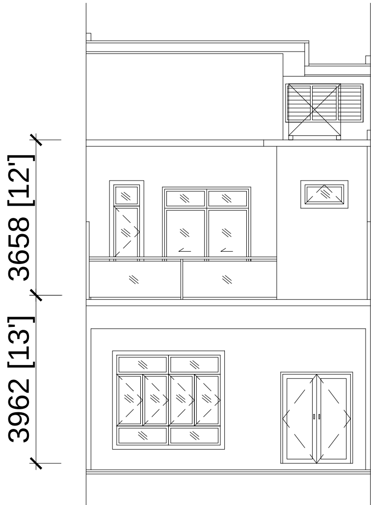
PANDANGAN HADAPAN RUMAH TERES 2 TINGKAT - TYPE B (PTD.4709,PTD.4711,PTD.4713,PTD.4715,PTD.4717,PTD.4719, PTD.4724,PTD.4726,PTD.4728,PTD.4730,PTD.4732,PTD.4734)
