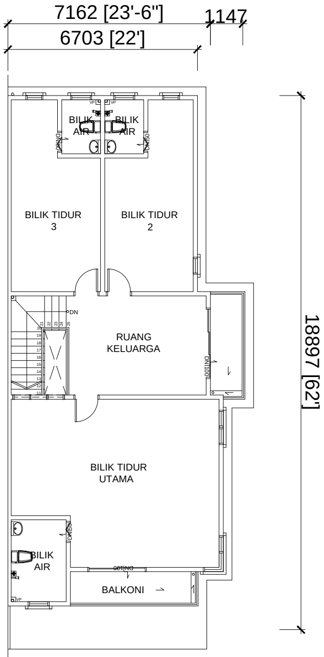
PELAN LANTAI TINGKAT ATAS RUMAH TERES 2 TINGKAT - TYPE D (PTD. 4707)
