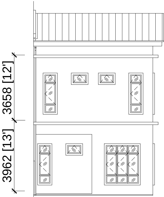
PANDANGAN BELAKANG RUMAH TERES 2 TINGKAT - TYPE C (PTD. 4720)
