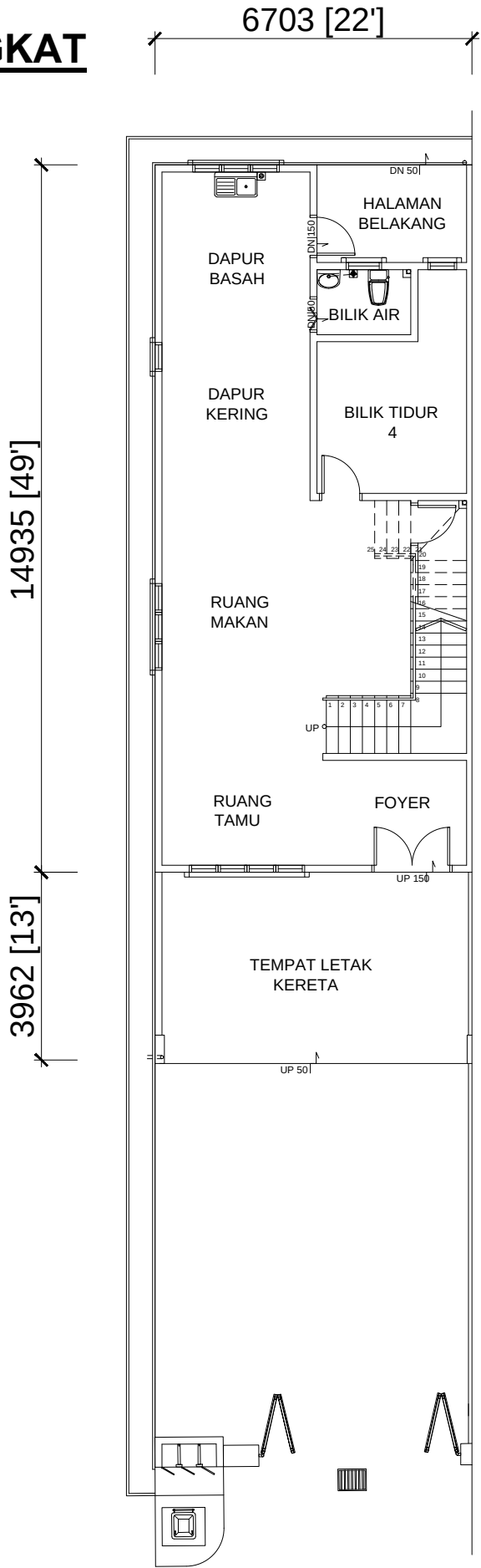
PELAN LANTAI BAWAH RUMAH TERES 2 TINGKAT - TYPE C (PTD. 4720)
