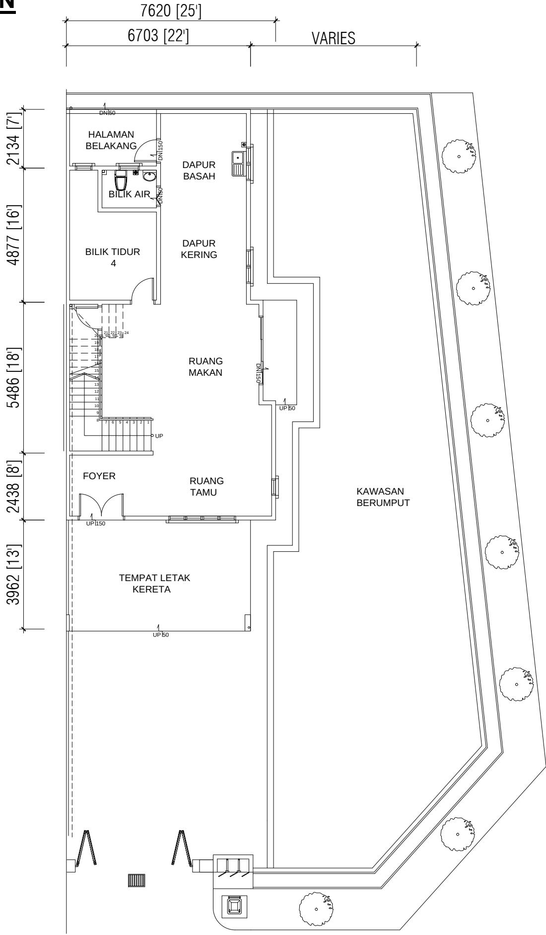
PELAN LANTAI BAWAH RUMAH TERES 2 TINGKAT - TYPE D (PTD. 4707)
