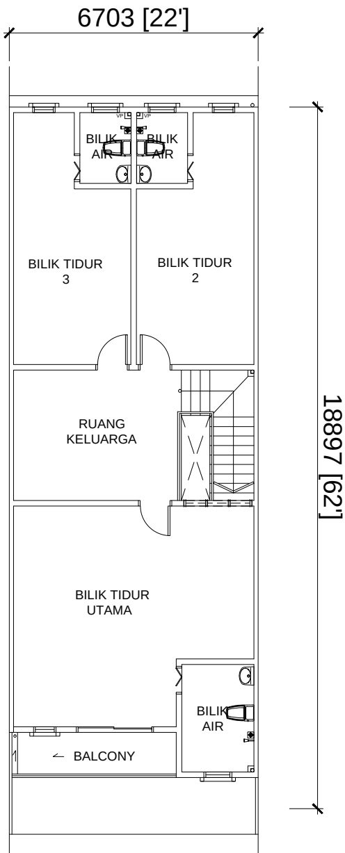
PELAN LANTAI TINGKAT ATAS RUMAH TERES 2 TINGKAT - TYPE B (PTD.4709,PTD.4711,PTD.4713,PTD.4715,PTD.4717,PTD.4719, PTD.4724,PTD.4726,PTD.4728,PTD.4730,PTD.4732,PTD.4734)
