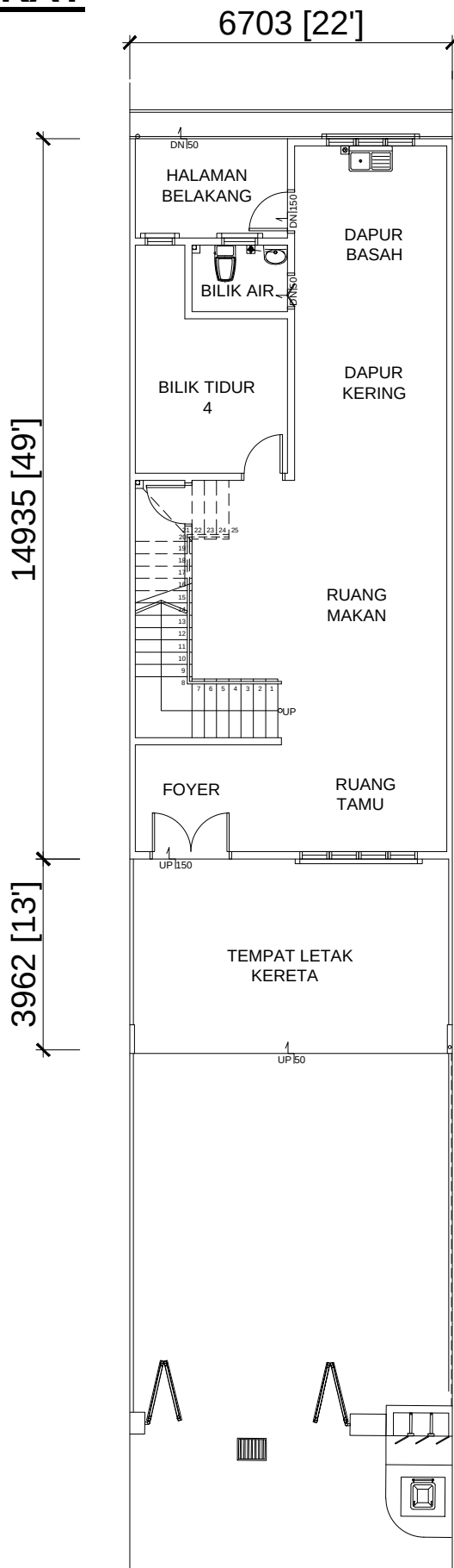
PELAN LANTAI BAWAH RUMAH TERES 2 TINGKAT - TYPE B (PTD.4708,PTD.4710,PTD.4712,PTD.4714,PTD.4716, PTD.4718,PTD.4723,PTD.4725,PTD.4727,PTD.4729, PTD.4731,PTD.4733)
