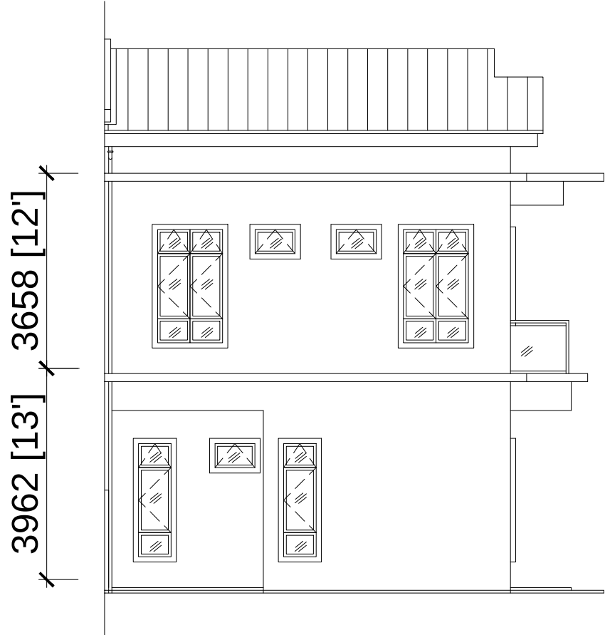
PANDANGAN BELAKANG RUMAH TERES 2 TINGKAT - TYPE A (PTD. 4722)
