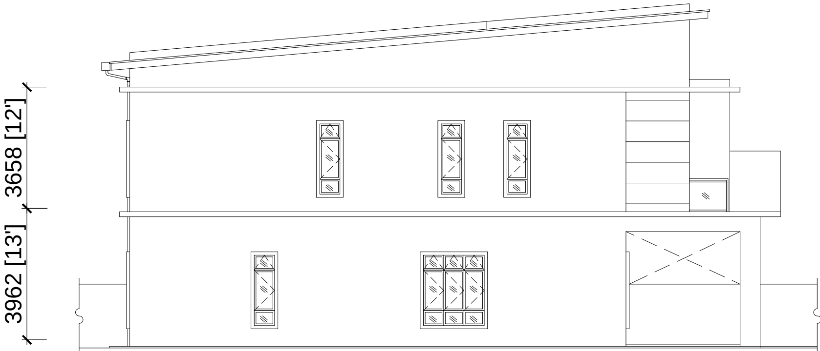
PANDANG SISI RUMAH TERES 2 TINGKAT - TYPE C (PTD. 4720)
