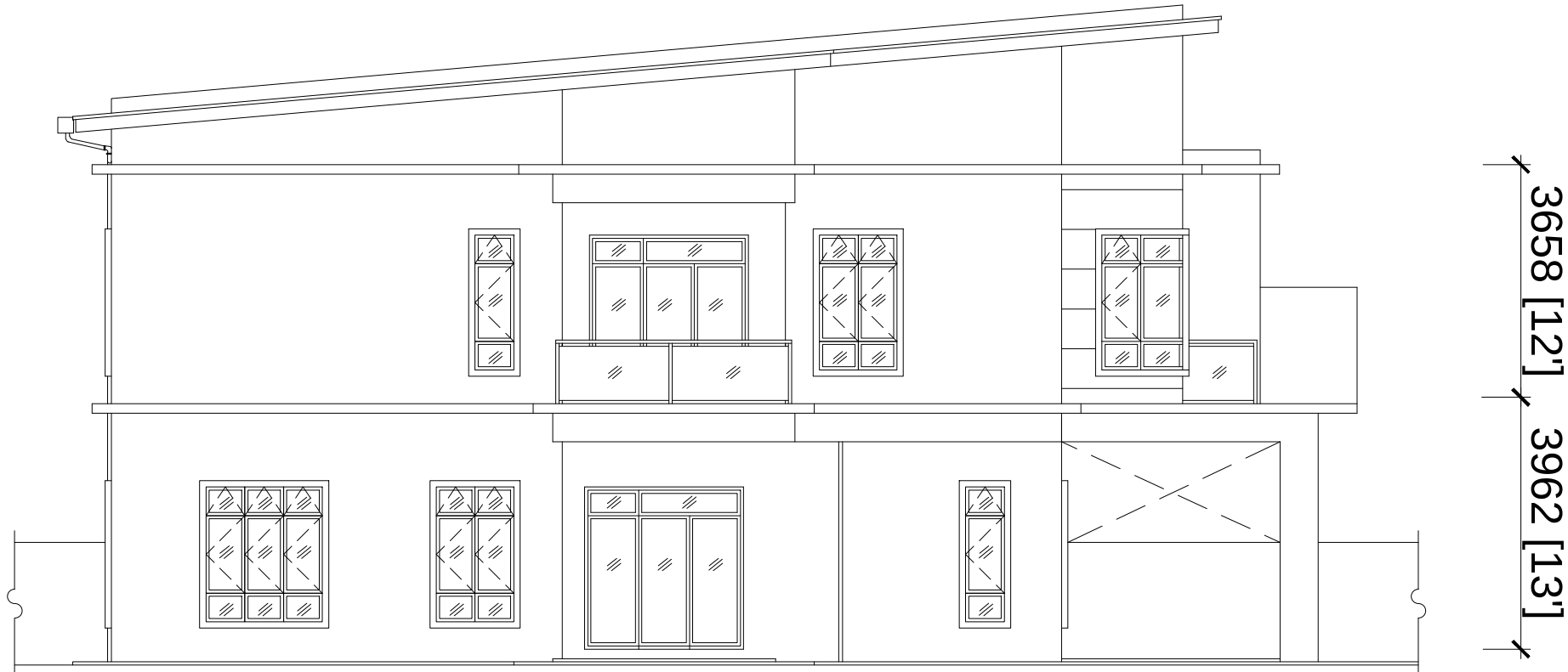
PANDANG SISI RUMAH TERES 2 TINGKAT - TYPE A (PTD. 4722)
