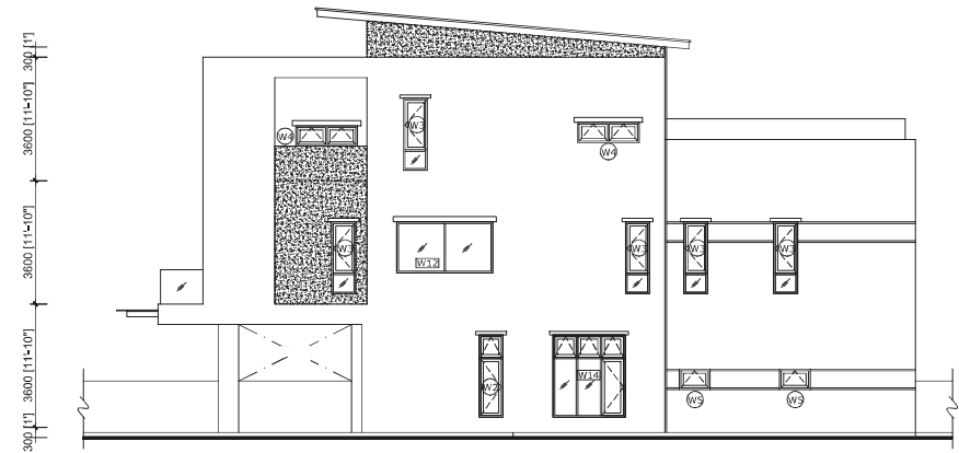
PELAN PANDANGAN KANAN BANGUNAN
