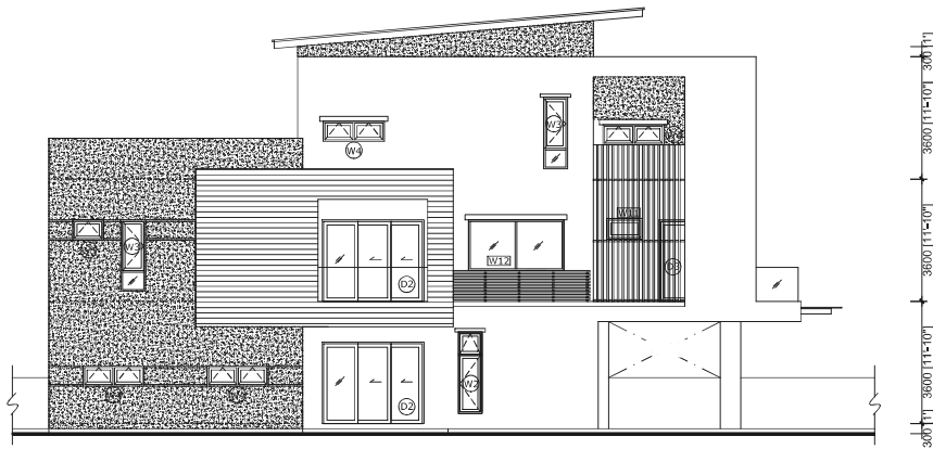
PELAN PANDANGAN KIRI BANGUNAN
