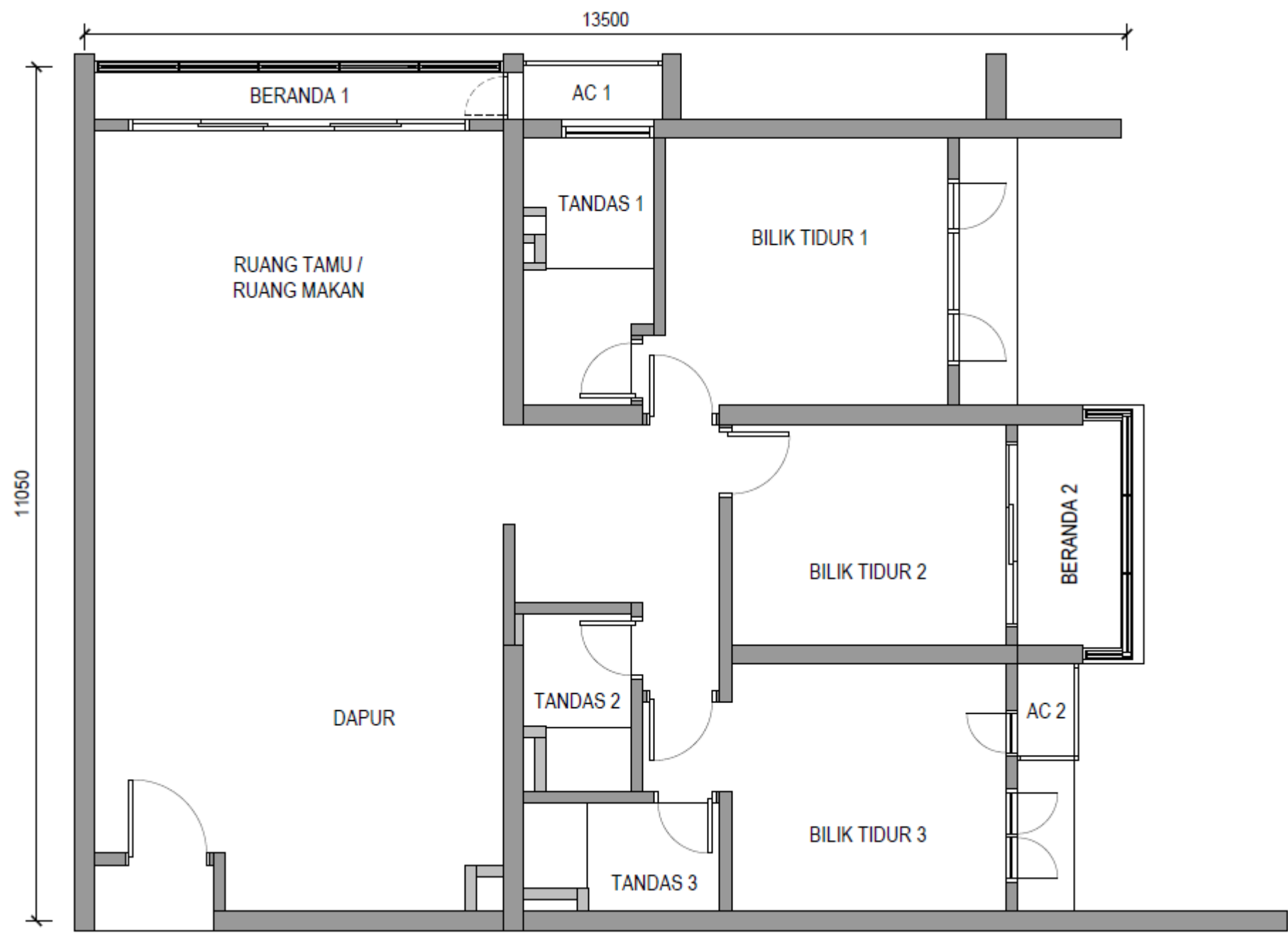
Pelan Lantai Jenis H2 - 1,422 kaki persegi (3unit)
