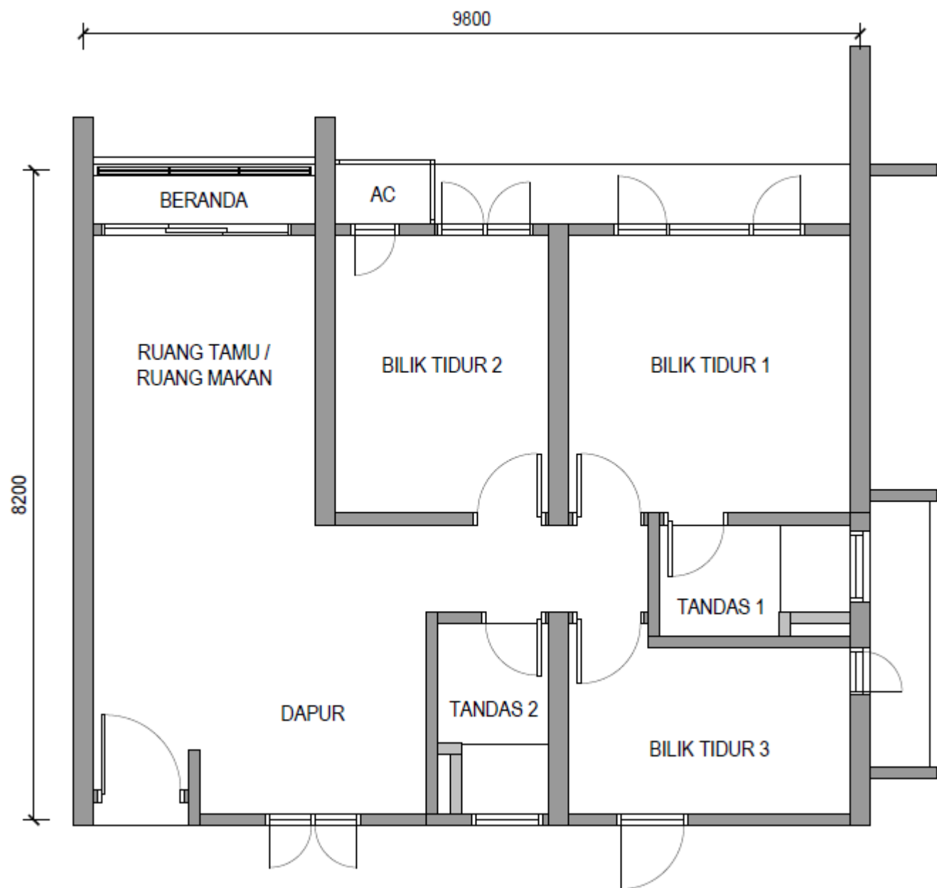
Pelan Lantai Jenis B2 - 822 kaki persegi (96 unit)
