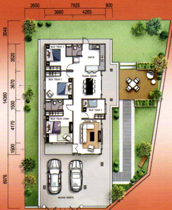
PELAN LANTAI RUMAH BANGLO 1 TINGKAT
