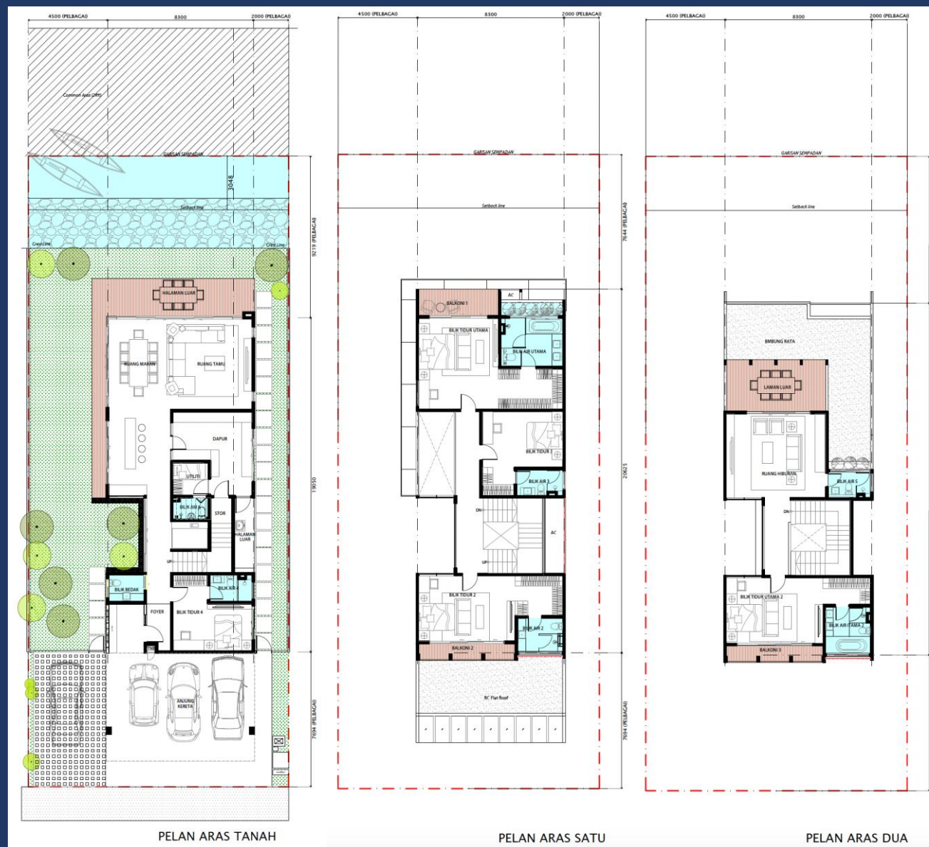
JENIS A1 – 4,914 k.p Pelan Aras Tanah, Aras 1 dan Aras 2
