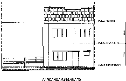
PANDANGAN BELAKANG
