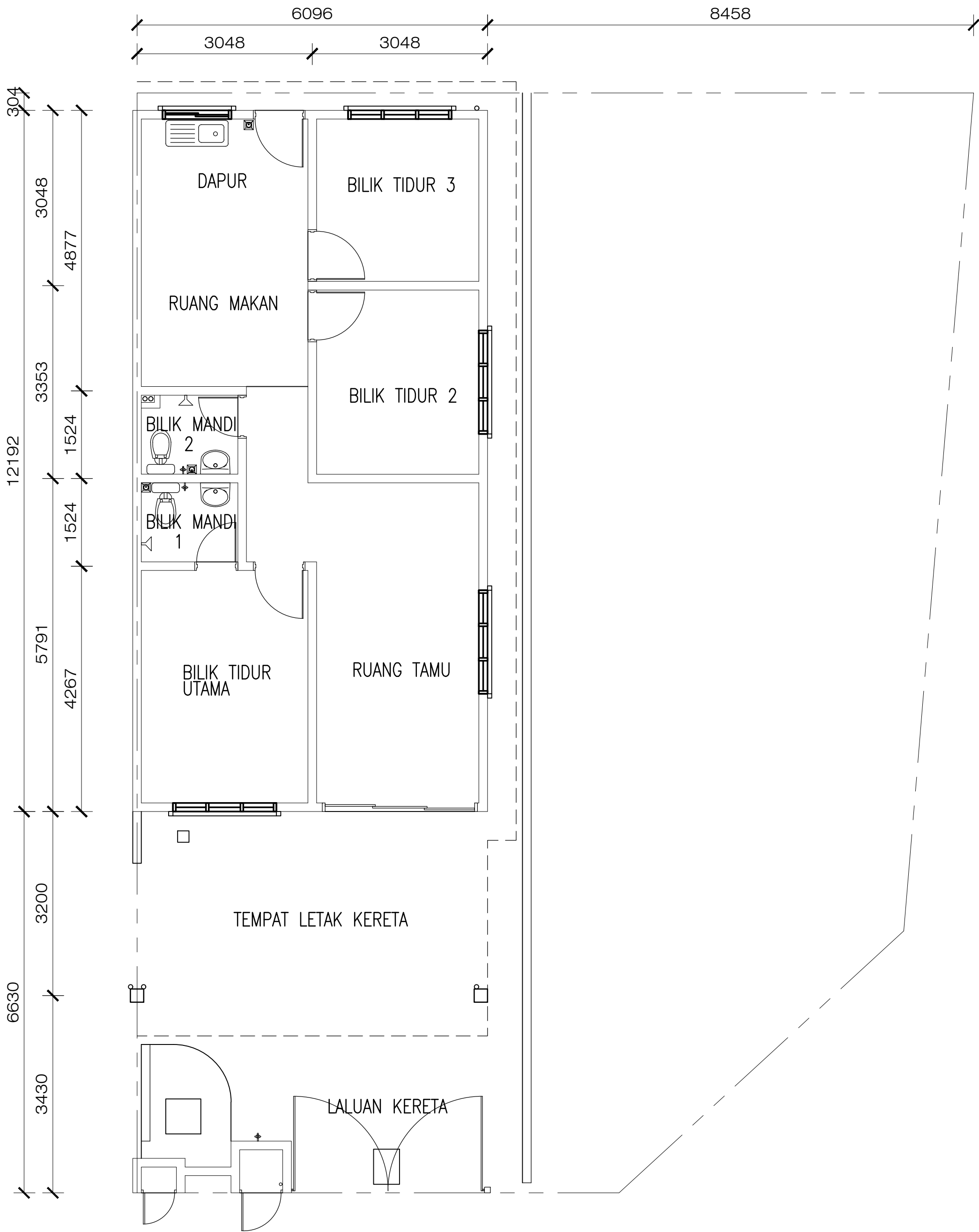
PELAN TINGKAT BAWAH
