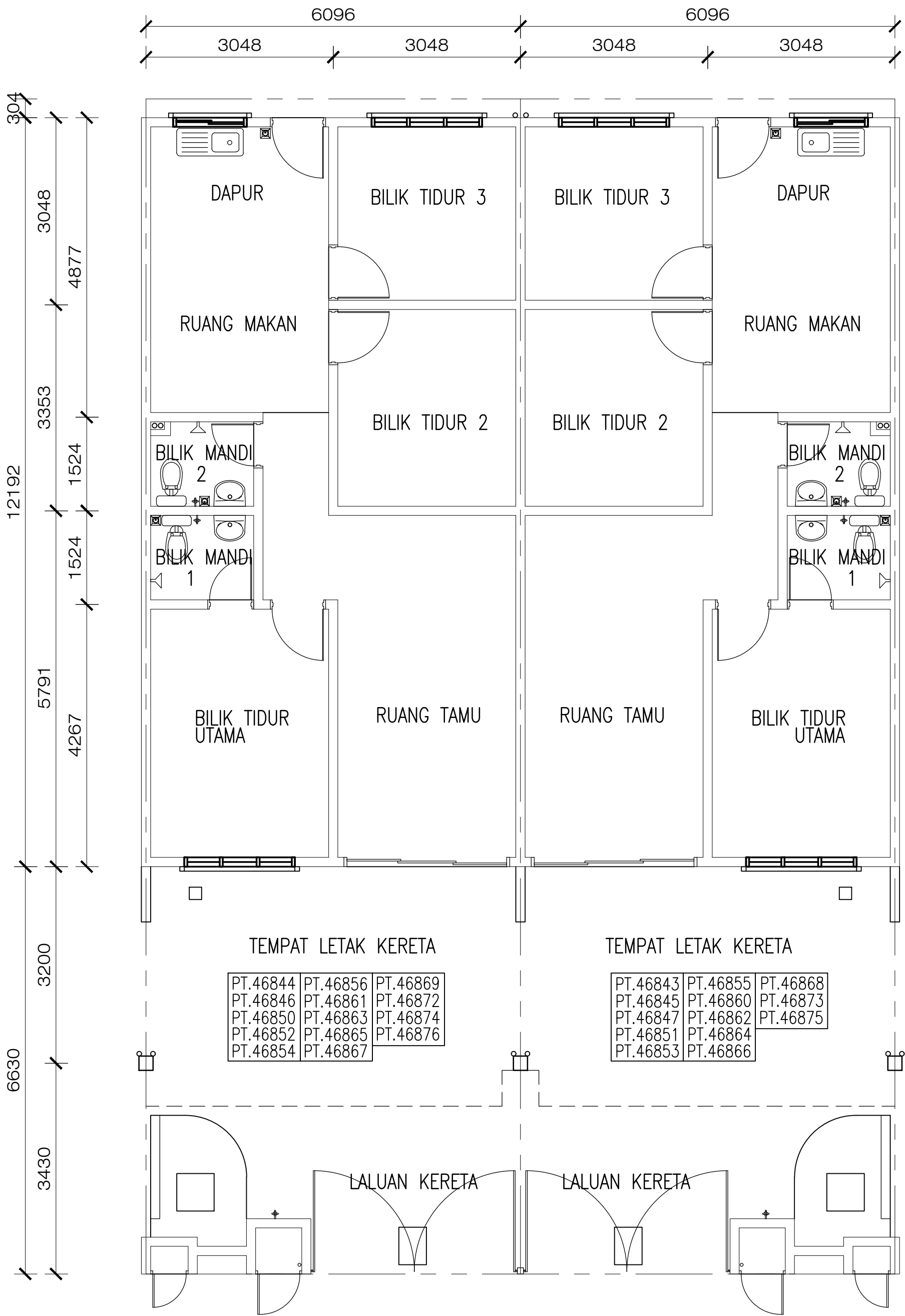
PELAN TINGKAT BAWAH
