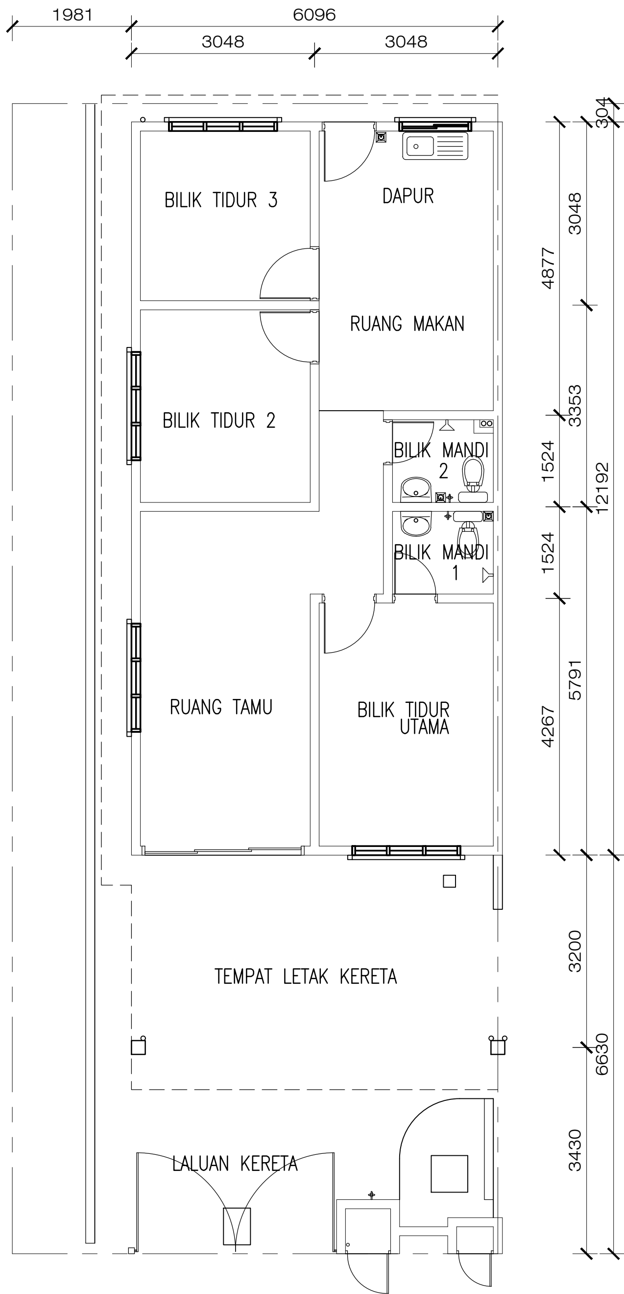
PELAN TINGKAT BAWAH
