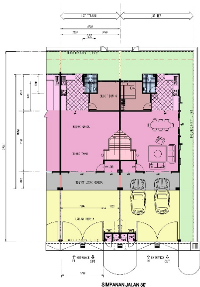
PELAN LANTAI TINGKAT TANAH
