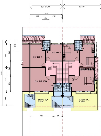
PELAN LANTAI TINGKAT SATU
