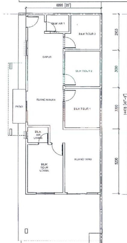
RUMAH KLUSTER 1 TINGKAT (30' X 67')
