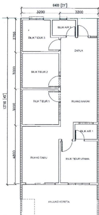
RUMAH TERES SATU TINGKAT (21' X 65')
