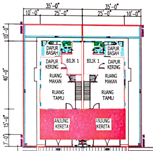
PELAN TINGKAT BAWAH
