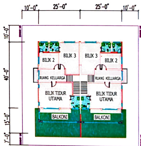
PELAN TINGKAT ATAS
