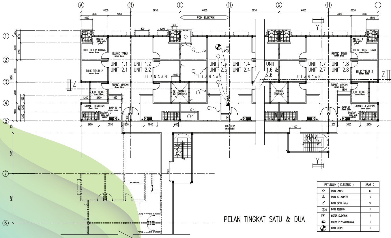
Pelan Tingkat 1 & 2
