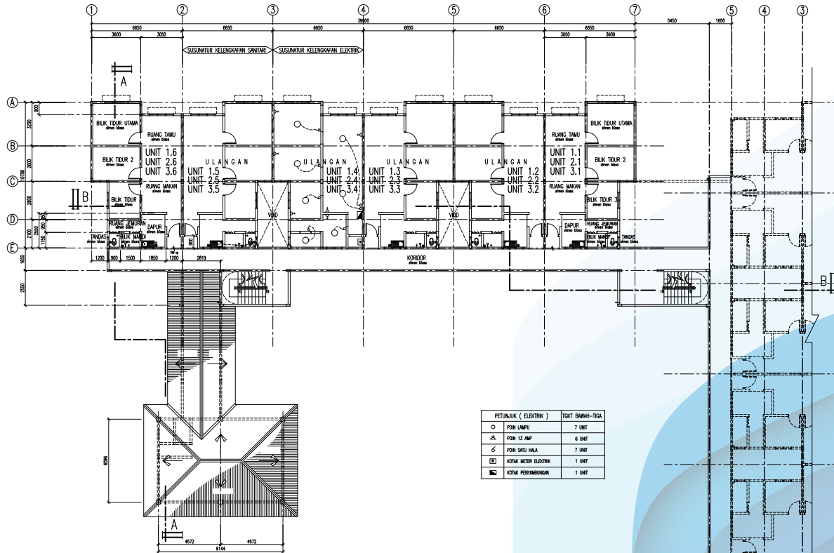
PELAN TINGKAT SATU – TINGKAT TIGA
