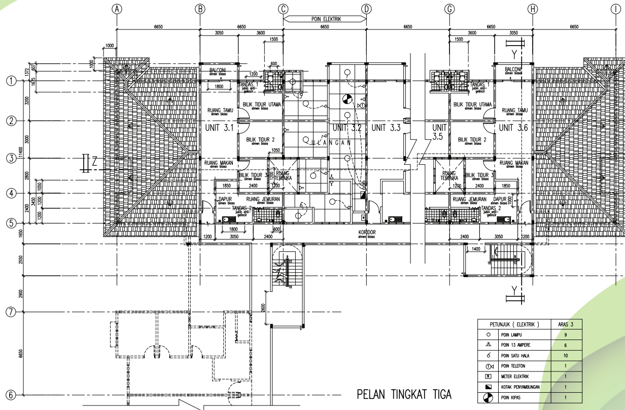
Pelan Tingkat 3
