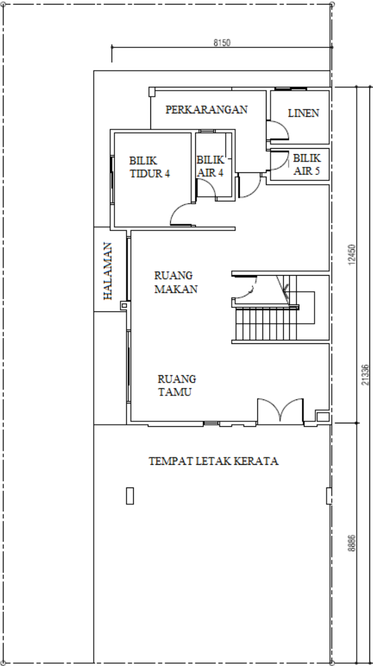
PELAN LANTAI TINGKAT BAWAH
