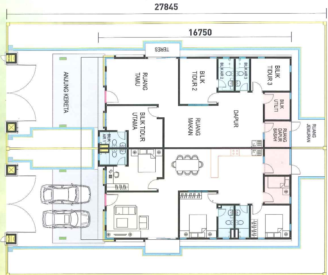
PELAN LANTAI
