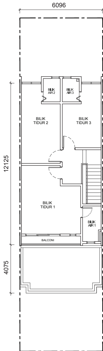
Tingkat Satu
