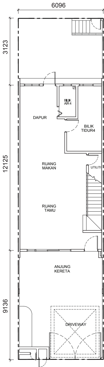
Tingkat Bawah
