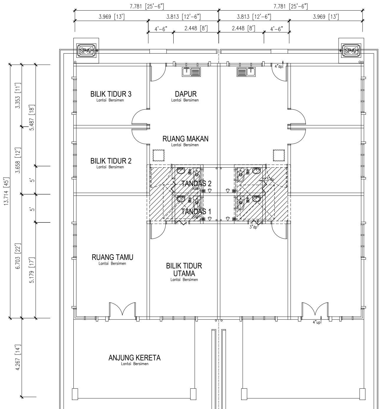
PELAN LANTAI
