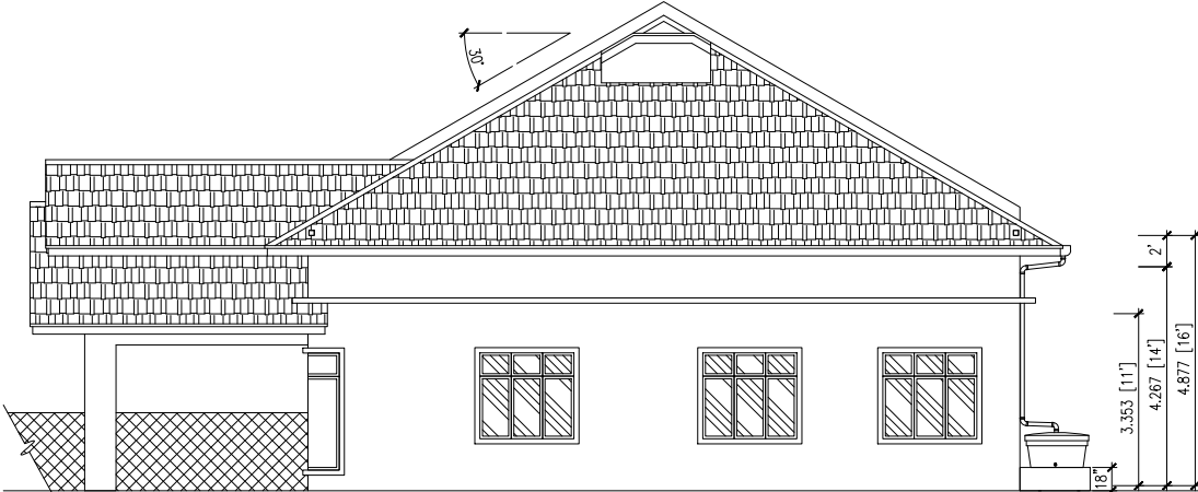
KANAN
