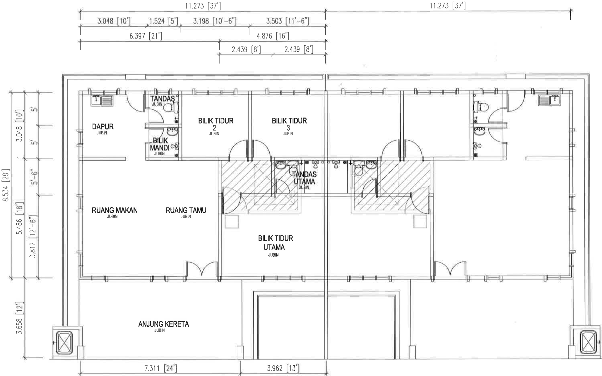
PELAN LANTAI
