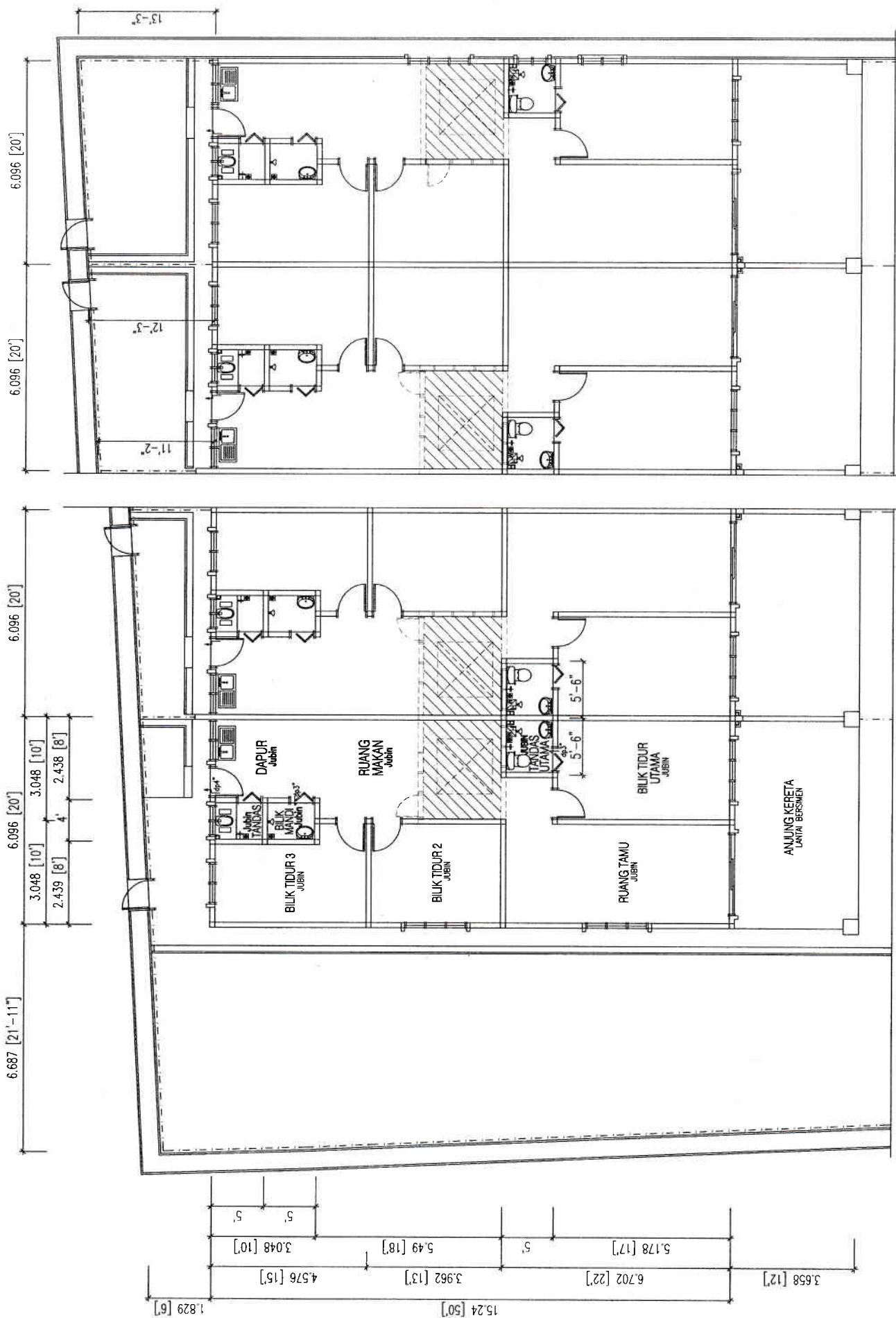
PELAN LANTAI
