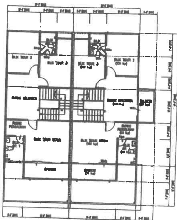
PELAN TINGKAT ATAS
