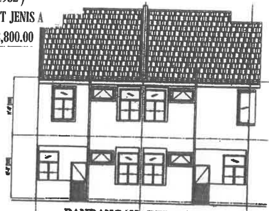
PANDANGAN BELAKANG
