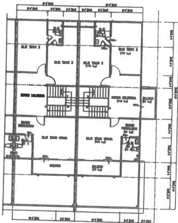
PELAN TINGKAT ATAS
