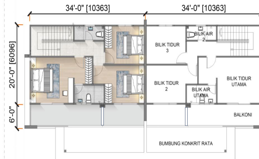
PELAN LANTAI TINGKAT ATAS TIPIKAL
