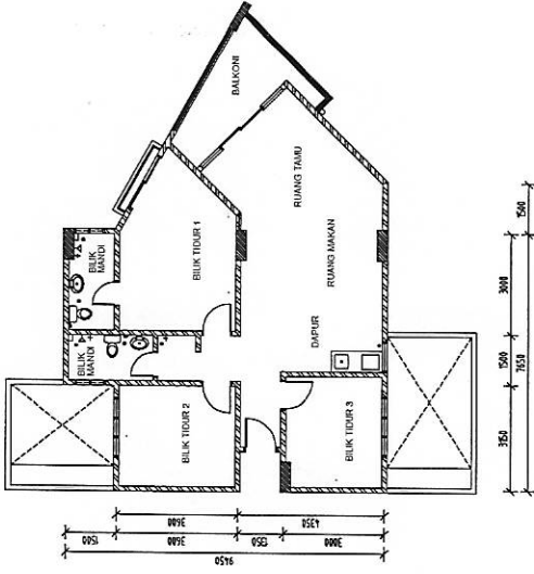
Jenis A 3 Bilik 1055 sf
