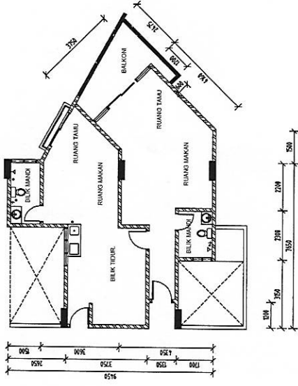
Jenis B - 2 Bilik 912 sf
