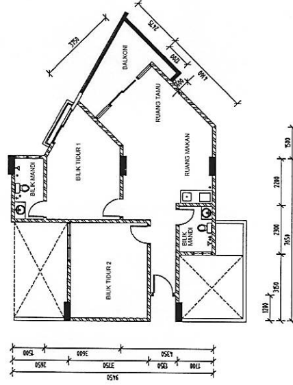
Jenis B1 - 2 Bilik 912 sf
