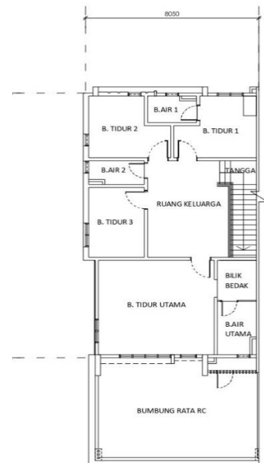
Pelan Lantai Tingkat Atas
