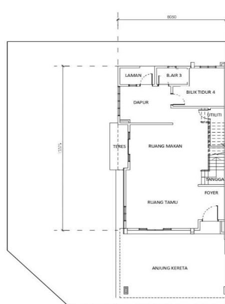
Pelan Lantai Tingkat Bawah
