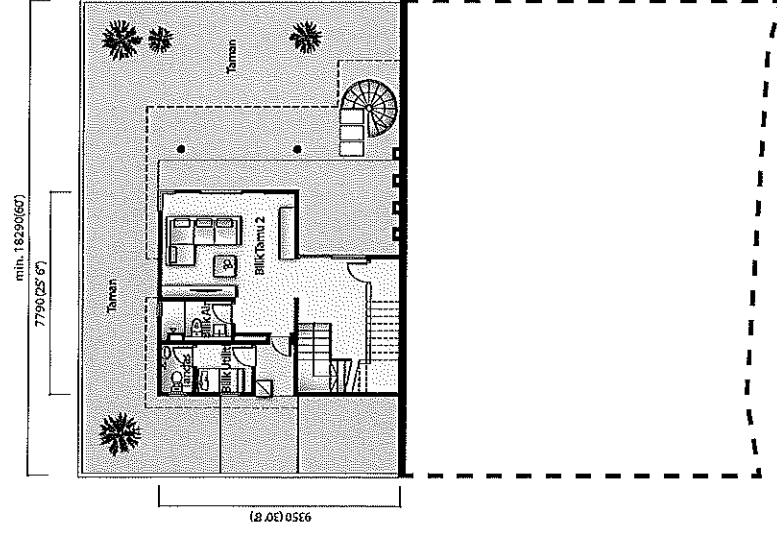
Pelan Tingkat Bawah Satu
