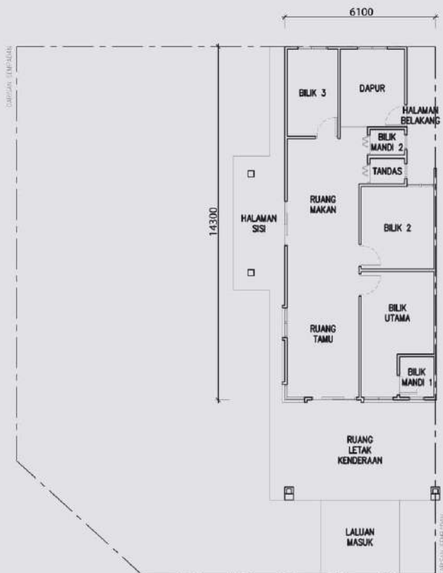
RUMAH TERES 1 TINGKAT (20' X 70')
